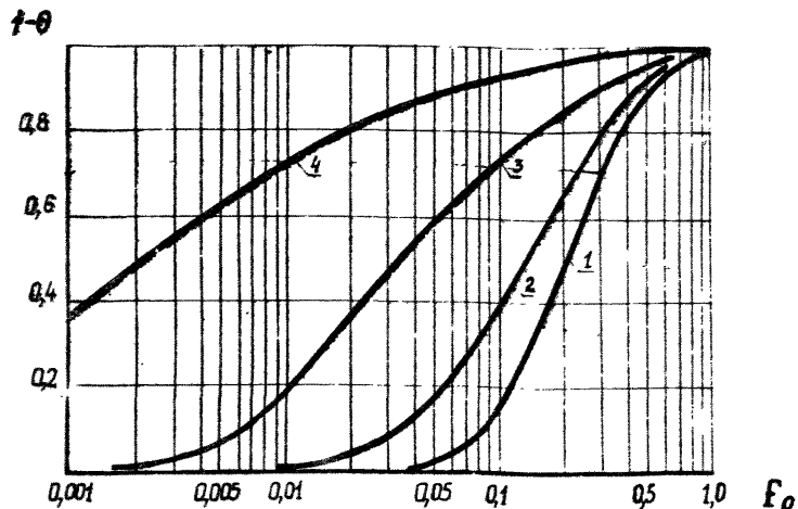
Рис. 6. Снижение безразмерной температуры для различных точек пласта во времени после обработки. 1-z=0 ; 2-z=0,5R ; 3-z=0,8R ; 4-z=0,95R , R - расчетное положение электроды (Т пл. +10°C) на момент отключения электронагревателя; F_0 - безразмерное время; F_0 = \frac{\lambda \tau}{C R^2} ; \lambda - коэффициент теплопроводности, \frac{\text{Вт}}{\text{м}^2 \text{град}} ; C - объемная теплоемкость, \frac{\text{Вт час}}{\text{м}^3 \text{град}} ; \tau - время с момента отключения электронагревателя, час; z - расстояние от оси скважины, м; Т пл. - температура плавления парафино-смолистых осадков, °C.
