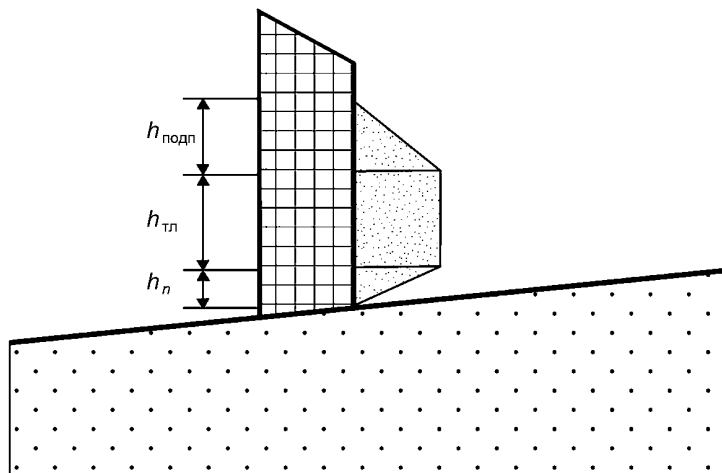
Рисунок Б.5 — Определение высоты подпора лавины h_{\text{подп}} необтекаемым препятствием
