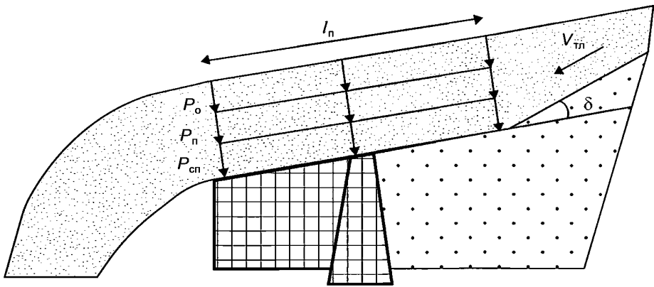
Рисунок Б.8 — Перетекание наклонной поверхности здания (галереи)
