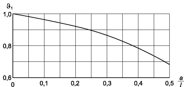
Рисунок 5.3 — Значения коэффициента \eta_1
