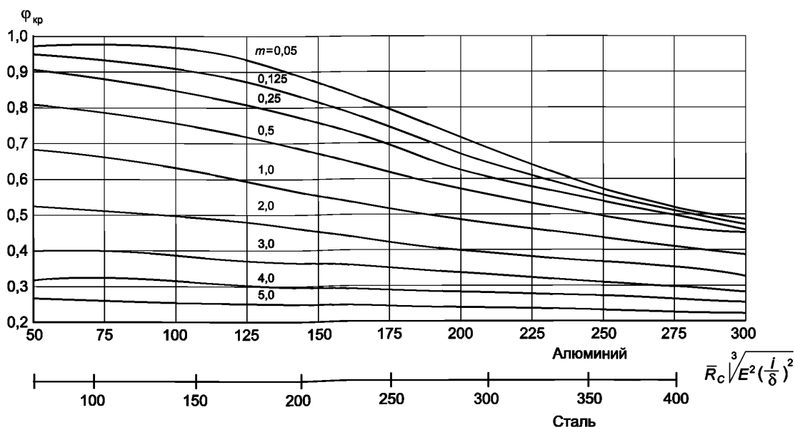
Рисунок 5.5 — График для определения \varphi_{\text{кр}}
