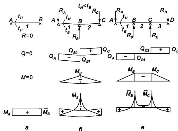
Рисунок 5.2 — Усилия в изгибаемой ограждающей однопролетной (а), двухпролетной (б), трехпролетной (в) конструкции
