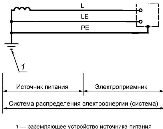
Рисунок 20.3 — Система распределения электроэнергии наименьшего размера
