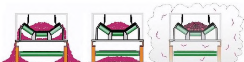
Просыпание угля Падение прилипшего угля с холостой ветви Попадание пыли в воздух при перегрузке Рисунок 57 – Пути попадания пыли в воздух при перемещении угля ленточным транспортером
