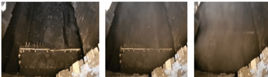
Рисунок 50 – Фазы работы дробильно-фрезерной машины. Организованный источник пыления
