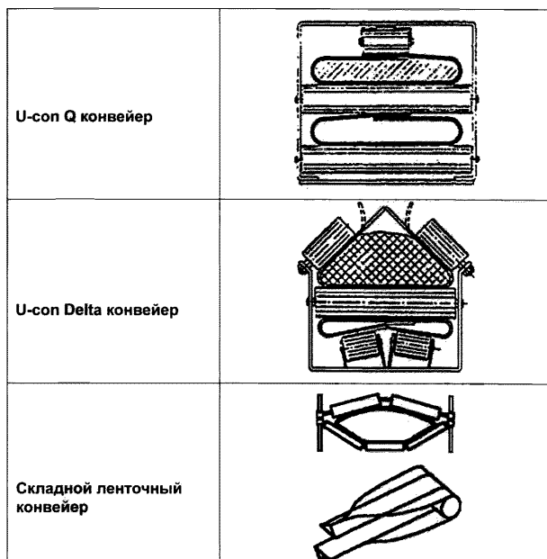
Рисунок 34 – Примеры конвейеров со складывающейся лентой
