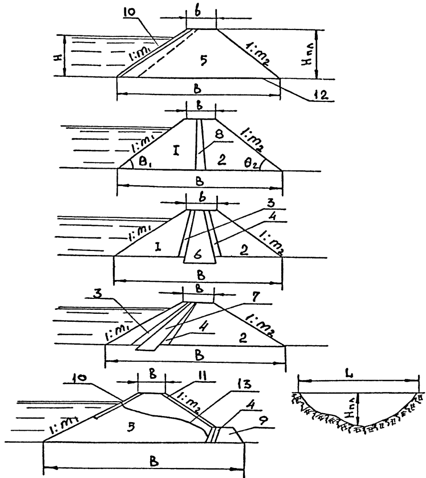
Рис.1 Основные элементы ограждающих дамб
