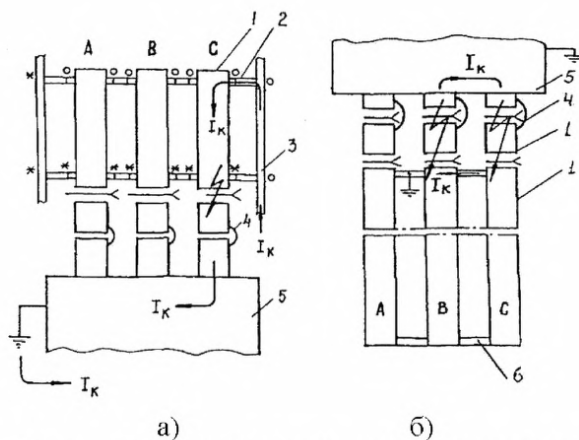
Рисунок В.1 – Схематичное изображение образования короткозамкнутого контура при нарушении изоляции:
