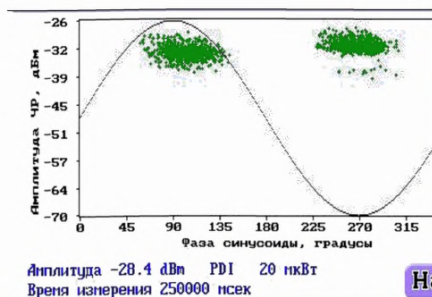
Рисунок Ж.9 – Типичное амплитудно-фазовое распределение интенсивности ЧР
