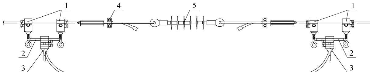
Вариант 2 ВЛЗ 6-20кВ
