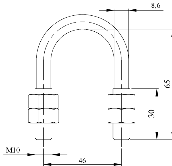
Хомут 1009889
