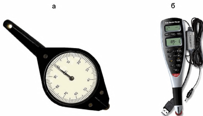
а – курвиметр механический КУ-А; б – курвиметр электронный «Scale Master Pro XE»
