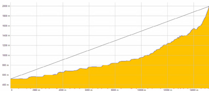
Рисунок В.4 – Продольный профиль реки Вердыз'рк
