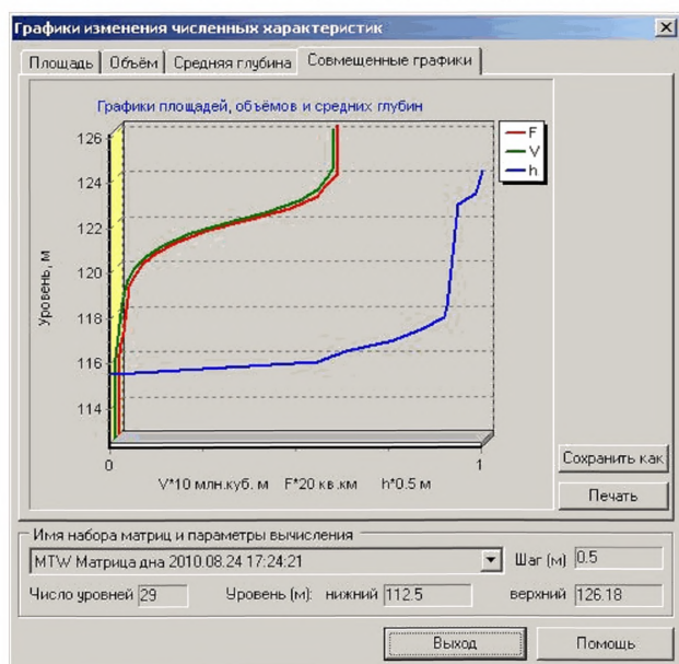
Рисунок 9.12 – Информационное окно графиков изменений численных характеристик водонаполнения
