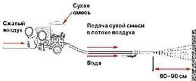
Рисунок 10.3 – Схема сухого способа пневмобетонирования (торкретирования)
