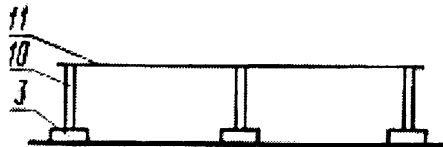
г) ограждения с доборными элементами
