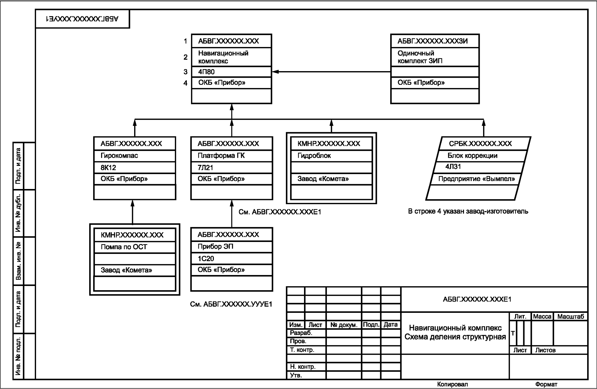
Рисунок Б.1 — Пример оформления схемы деления изделия при выполнении в бумажной форме
