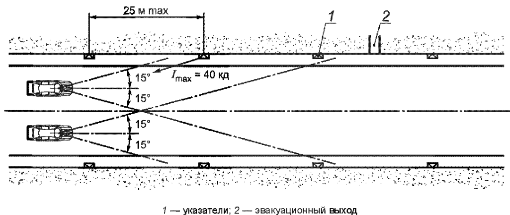
Рисунок 9.1 — Области ограничения слепящего действия указателей направления эвакуации
