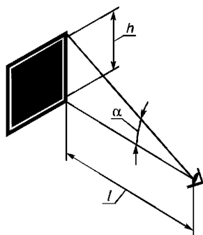
Рисунок 7.1 — Расчет высоты знака безопасности
