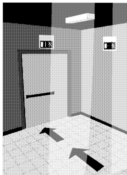
Рисунок 5.6 — Расположение светильника эвакуационного освещения в местах расположения знаков безопасности
