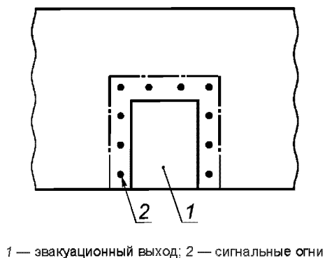
Рисунок 9.2 — Пример расположения сигнальных огней относительно эвакуационного выхода
