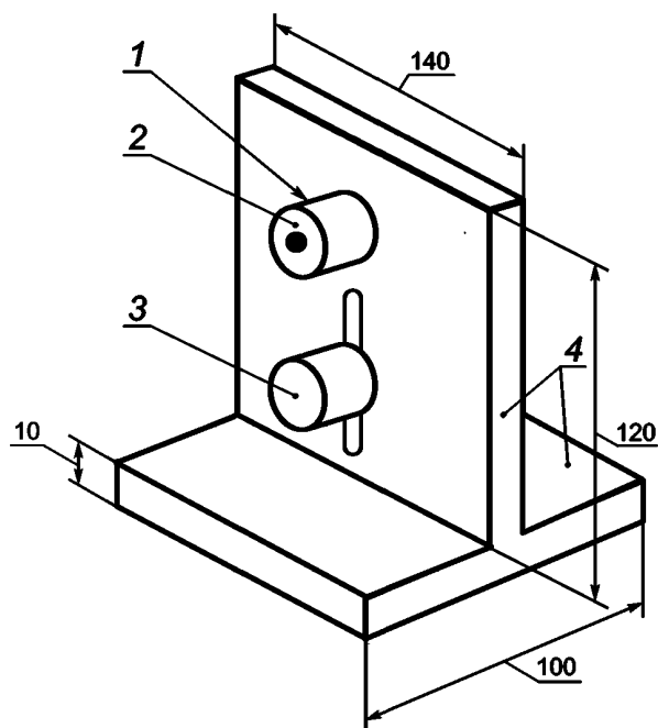
1а — Стенд для испытания манжет
