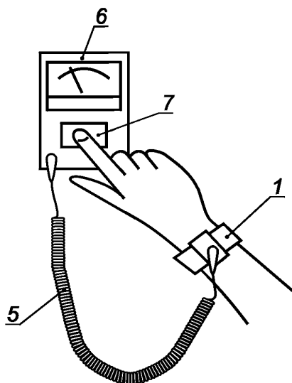
3б — Испытания с использованием специального устройства контроля
