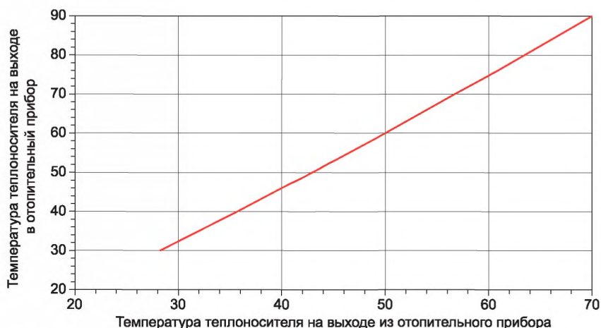
Рисунок 1 — Температура теплоносителя на входе и выходе из отопительного прибора при базовом расходе теплоносителя и t_{L,B} плюс 20 °С
