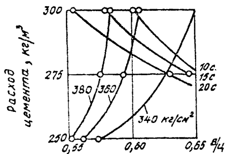
Рис. 3. Зависимость времени прохождения бетонной смеси по лотку при вибрировании от водоцементного отношения (а) и расхода цемента (б). песок M_K=1,0 ; цемент М 500
