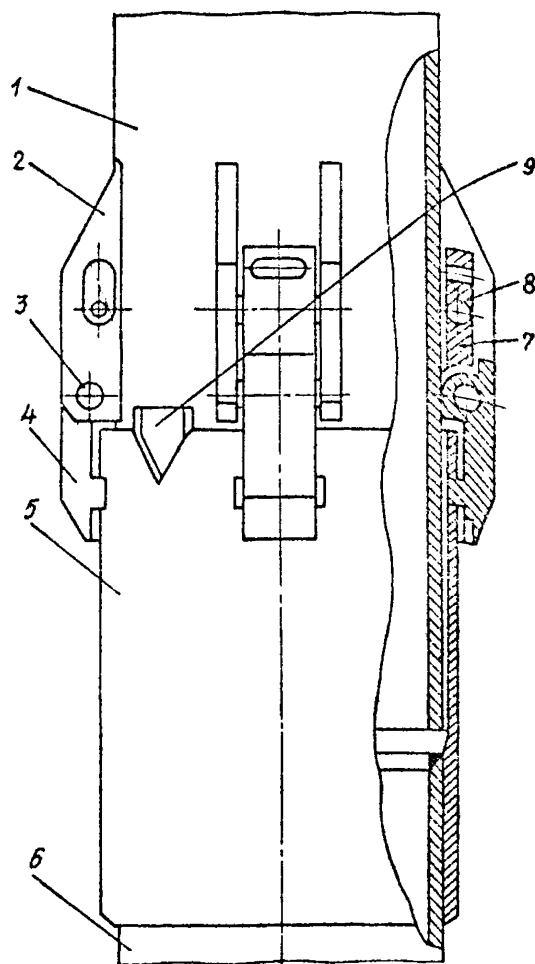
Рис. 6. Схема секции сборной бетонной трубы конструкции треста Укогидрострой: 1-нижний конец секции; 2-щека; 3-палец; 4-защелка, 5-раструб; 6-верхний конец секции; 7-фиксирующий ползун; 8-цапфа; 9-направляющая планка
