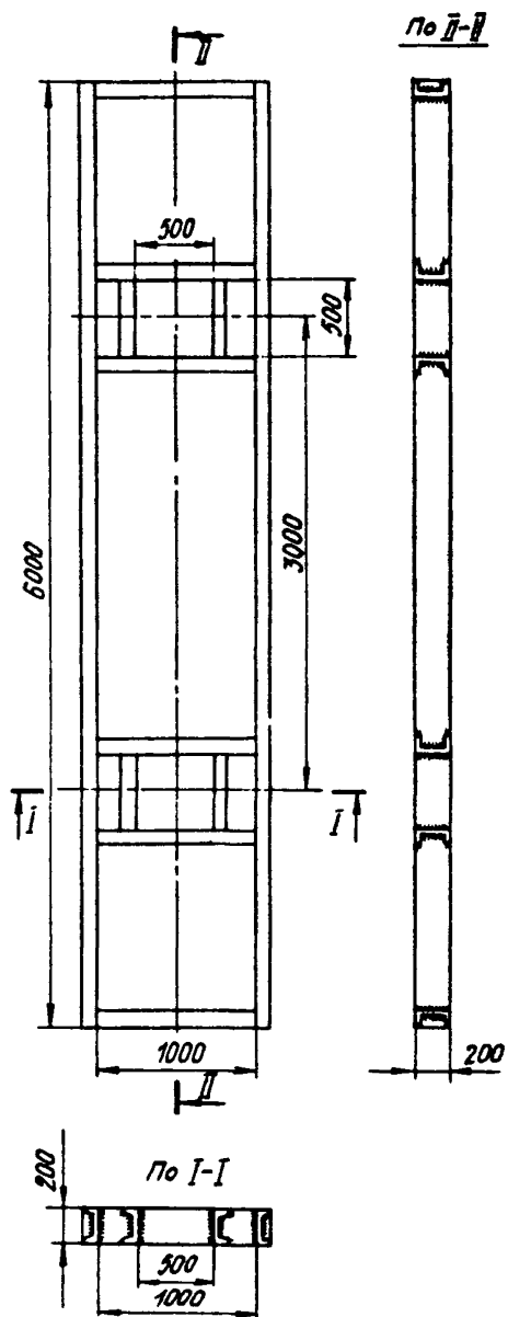
Рис. 3. Конструктивный вариант для фиксирования положения бетонных труб
