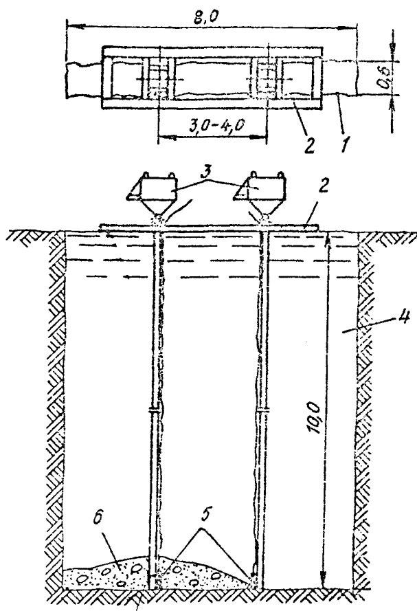
Рис. 13. Схема бетонирования захватки длиной 8 м двумя бетонолитными трубами: 1-траншея; 2-кондуктор; 3-бетонолитные трубы; 4-глинистый раствор; 5-вибраторы; 6-бетон
