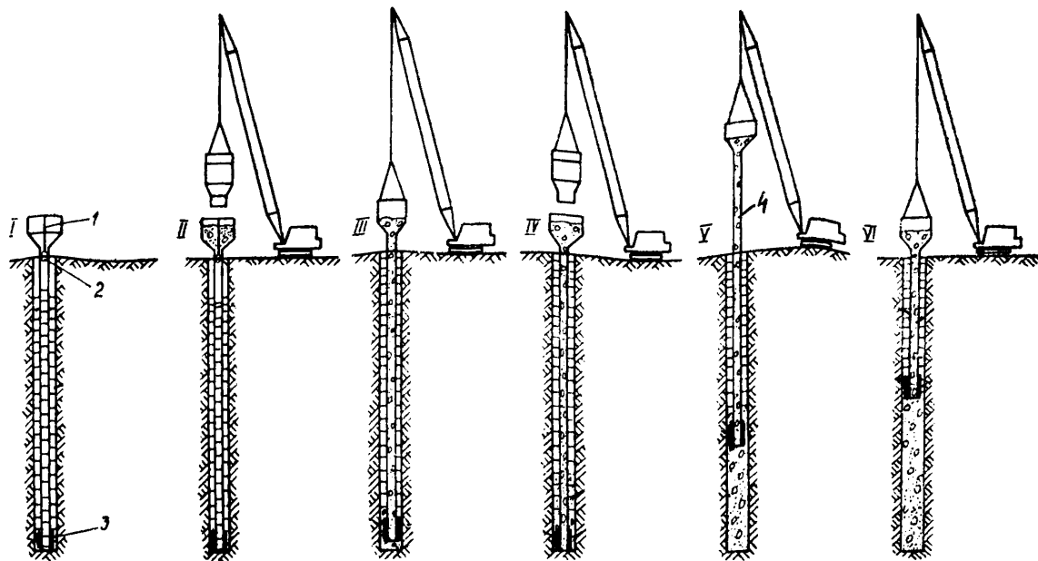
Рис. 14. Последовательность операций при бетонировании свай-оболочек бетонной смесью с вибрированием: I—установка на забой бетонной трубы с подвешенной скользящей пробкой; II—заполнение приемной воронки бетонной смесью; III—пуск первой порции бетона — труба приподнята над забоем; IV—заполнение приемной воронки второй и последующими порциями бетона; V—процесс бетонирования — труба приподнята на высоту подъема гака стрелы крана; VI—бетонирование после изъятия обжимной трубы; 1—подвес пробки; 2—стальная скользящая пробка; 3—вибратор
