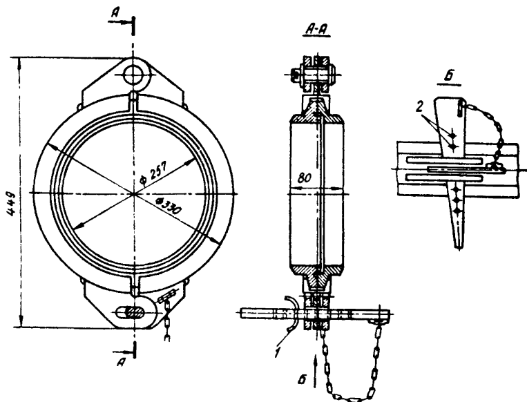
Рис. 5. Быстроразъемное соединение звеньев бетонной трубы: 1—шпилька; 2—отверстие диаметром 8 мм под шпильку
