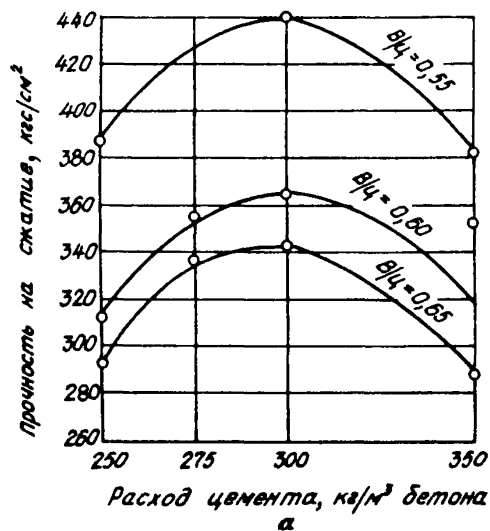
Рис. 2. Зависимость прочности бетона на песке M_{II}=I,0 : а-от расхода цемента; б-от цементно-водного отношения. Возраст бетона 180 суток
