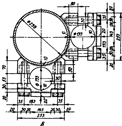
Рис. 9. Конструктивный вариант жесткого крепления вибратора ИВ-60 (С-826) к бетонолитной трубе: б — при глубинах бетонирования от 20 до 50 м
