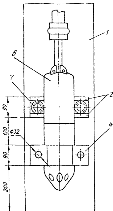
Рис. 9. Конструктивный вариант жесткого крепления вибратора ИВ-60 (С-826) к бетонолитной трубе: а - при глубинах бетонирования до 20 м; 1 - бетонолитная труба; 2 - подкладка; 3 - накладка; 4 - натяжной болт; 5 - отверстие под шпиль; 6 - вибратор; 7 - вкладыш диаметром 50 мм, высотой 50 мм
