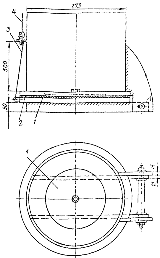
Рис. 12. Схема устройства донного клапана конструкции греста Гидроспецфундаментстрой: 1-прижимная шайба; 2-резьбовая прокладка; 3-веревка диаметром 4-8 мм; 4-грест диаметром 5-11 мм
