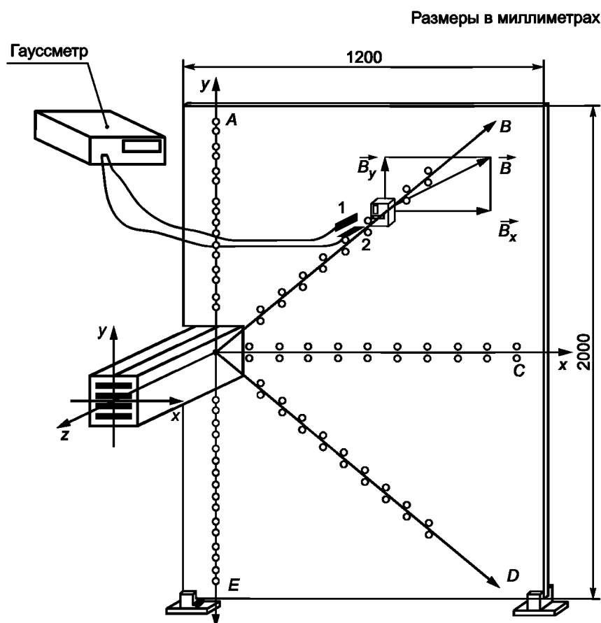
Рисунок ЕЕ.1 — Устройство для измерения магнитного поля
