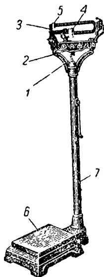
Рис. 9. Весы для взвешивания взрослых людей
