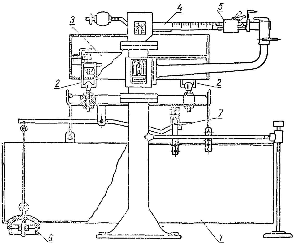
Рис. 11. Весы для жидкостей
