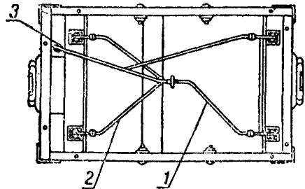
Рис. 4—5. Весы сотенные с качающейся платформой и коромыслом, опирающимся на стойку
