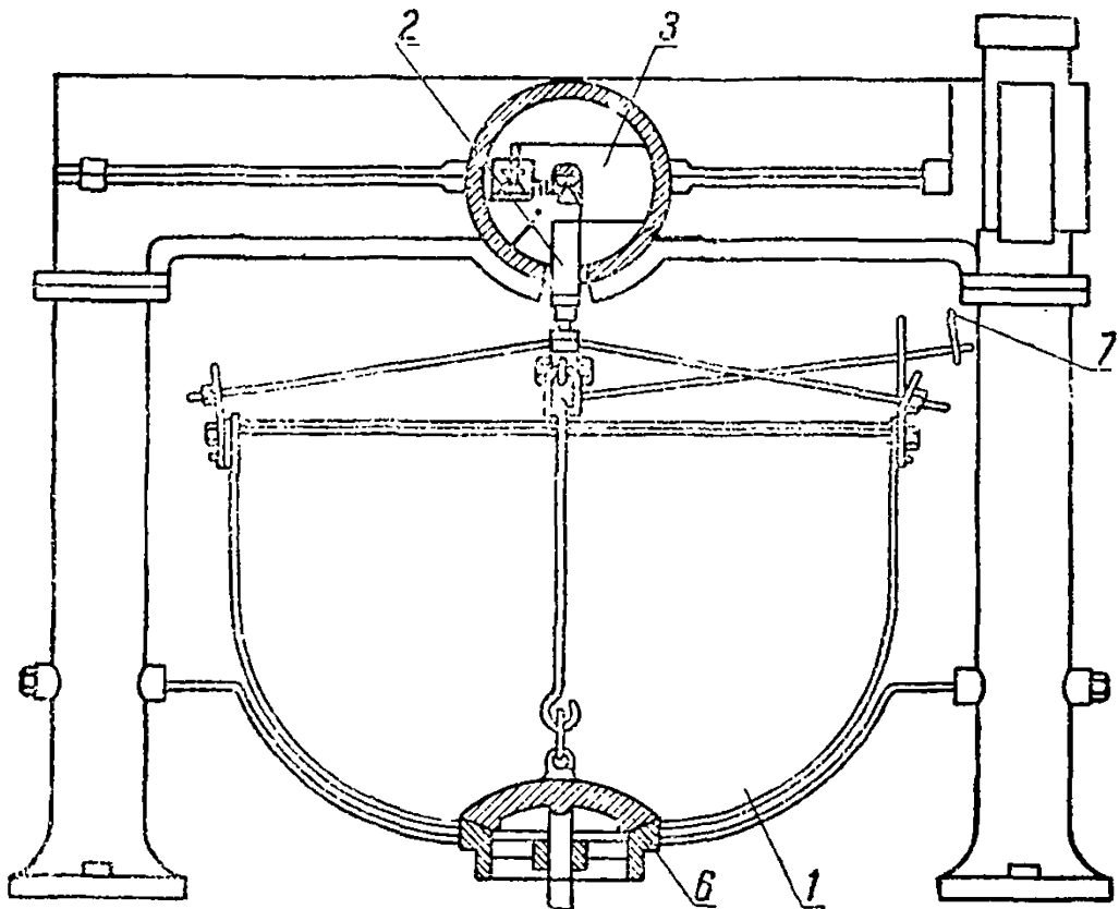
Рис. 12. Весы для жидкостей
