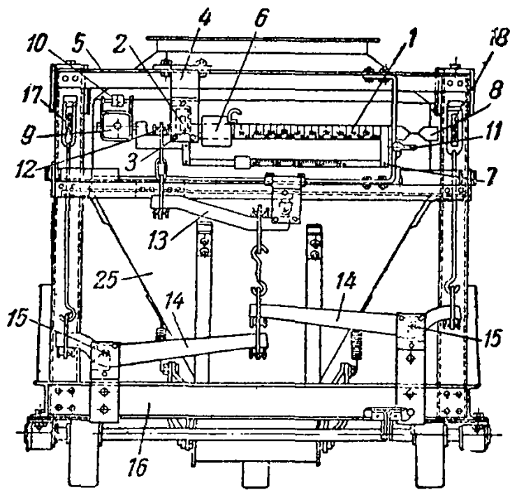
Рис. 14. Весы на тележке
