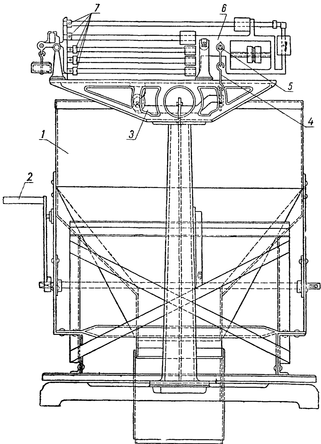
Рис. 13. Весы для шихты многошкальные
