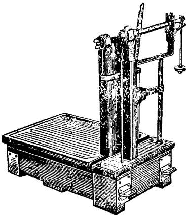
Рис. 4—5. Весы сотенные с качающейся платформой и коромыслом, опирающимся на стойку
