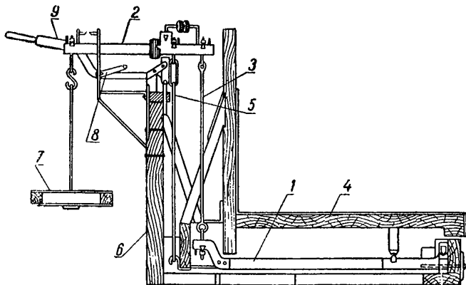
Рис. 1. Весы десятичные
