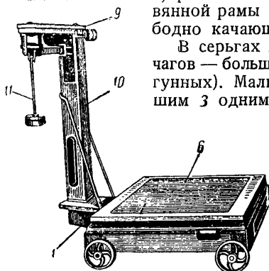
Рис. 2. Весы сотенные с качающимися рычагами и коромыслом, подвешенным на серьге
