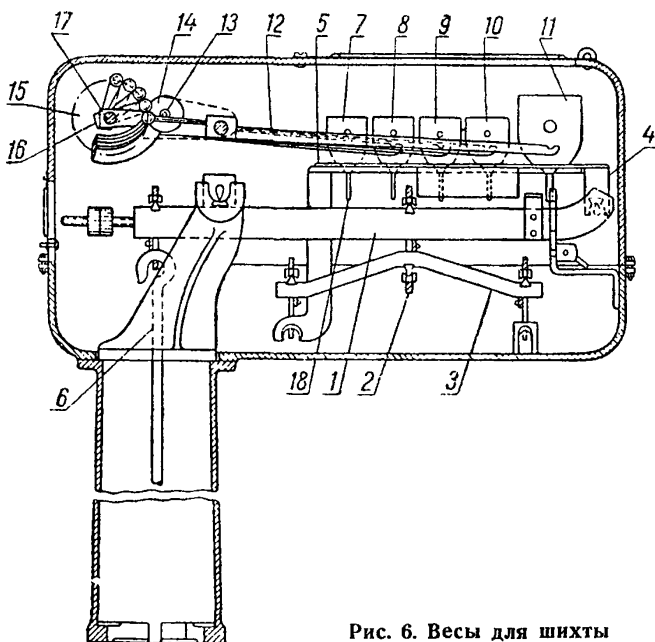
Рис. 6. Весы для шихты
