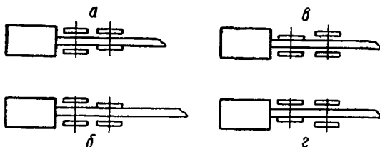
Рис. 17. Положения призм на подушках
