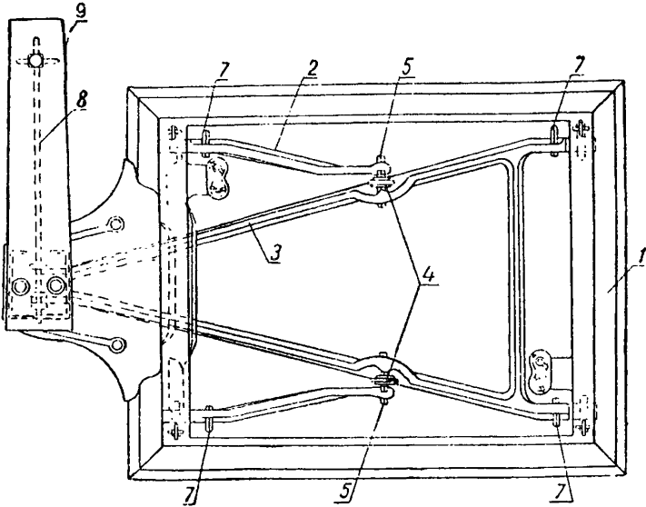
Рис. 3. Весы сотенные с качающимися рычагами и коромыслом, подвешенным на серьге
