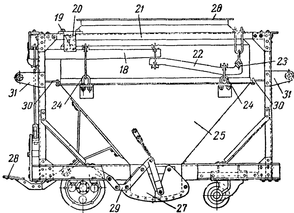
Рис. 15. Весы на тележке
