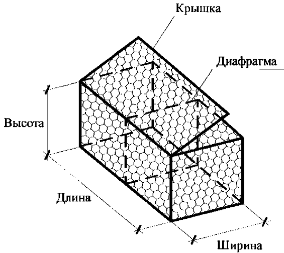
Рисунок 11 – Конструктивная схема габионных конструкций коробчатой формы
