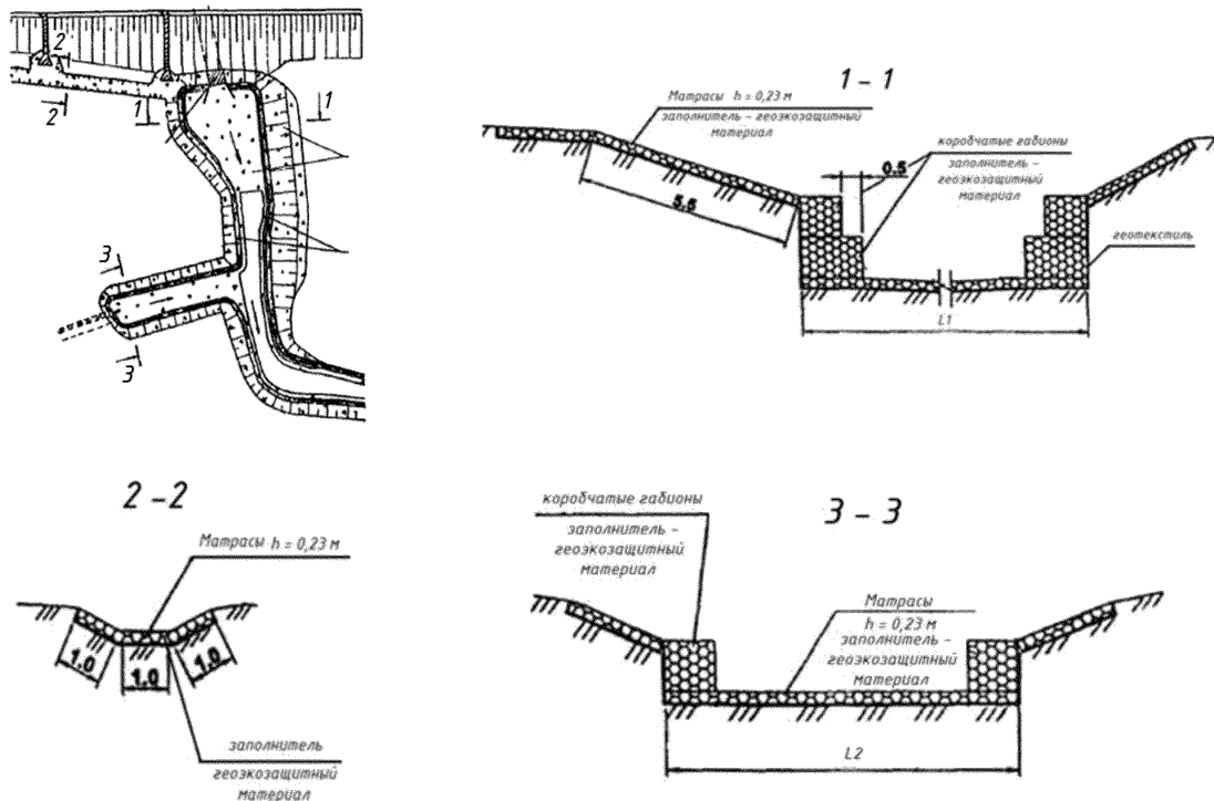
Рисунок 5 – Схема размещения и конструктивные особенности придорожного очистного сооружения из габионов
