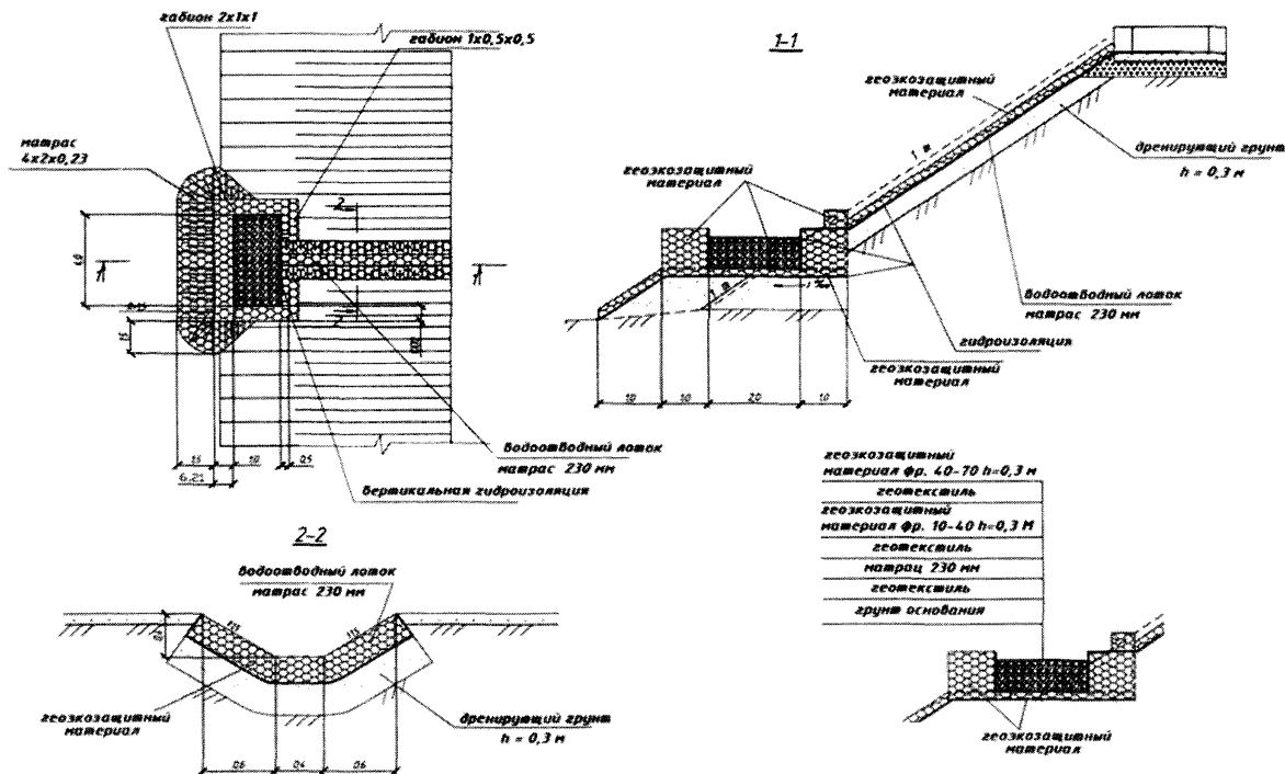
Рисунок 4 – Схема размещения геоэрозационных материалов для очистки поверхностных вод, собираемых с проезжей части автомобильных дорог
