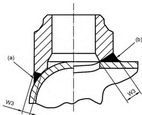
Рисунок 9.14.4-2 – Приварные штуцеры
