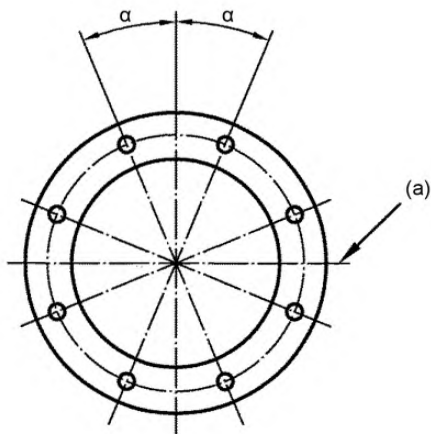
а – ось симметрии α – размер равномерно расположенных отверстий
