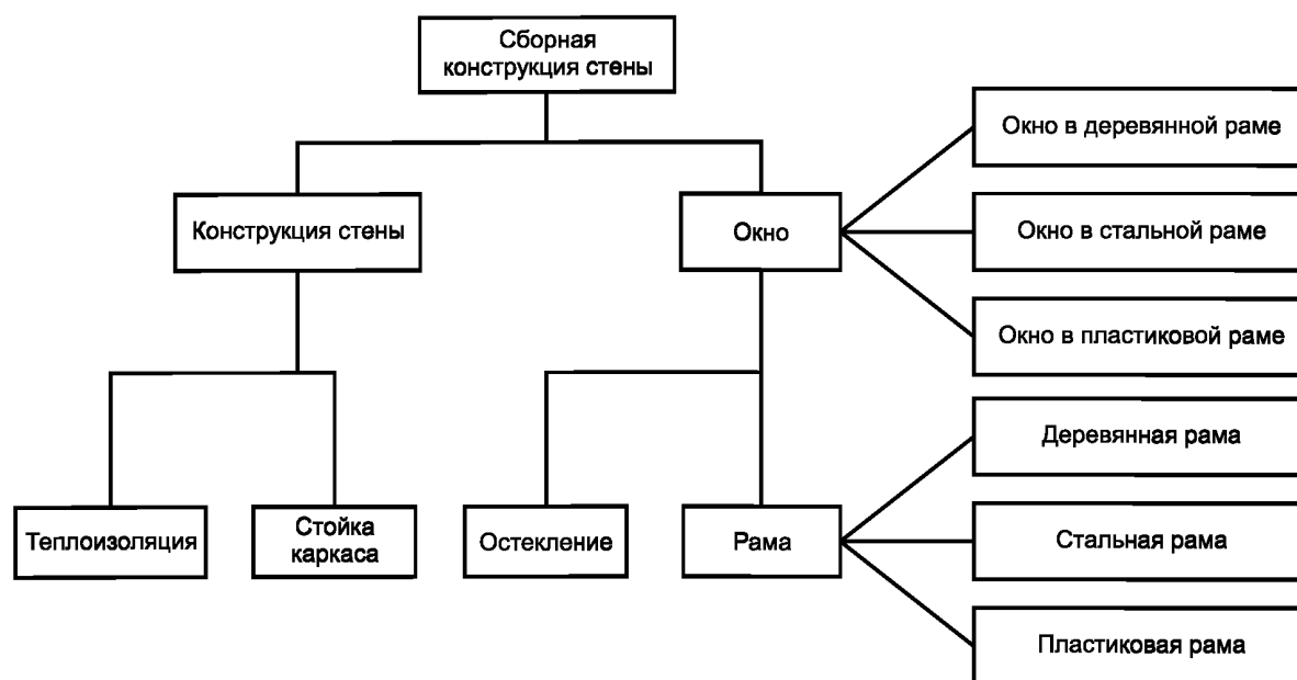
Рисунок 3 — Иллюстрация объединения композиции и классификации
