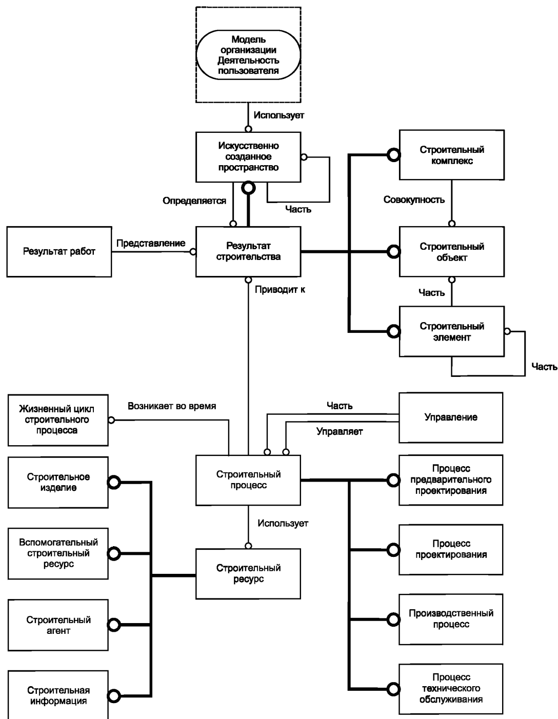
Рисунок 1 — Классы и их основные взаимосвязи
