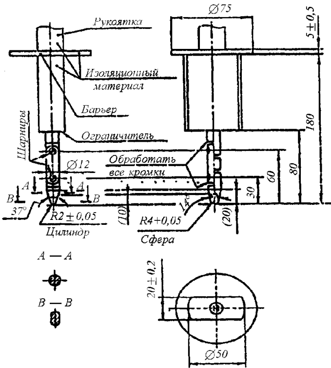
Рис. 5.1-1 Испытательный шарнирный палец
