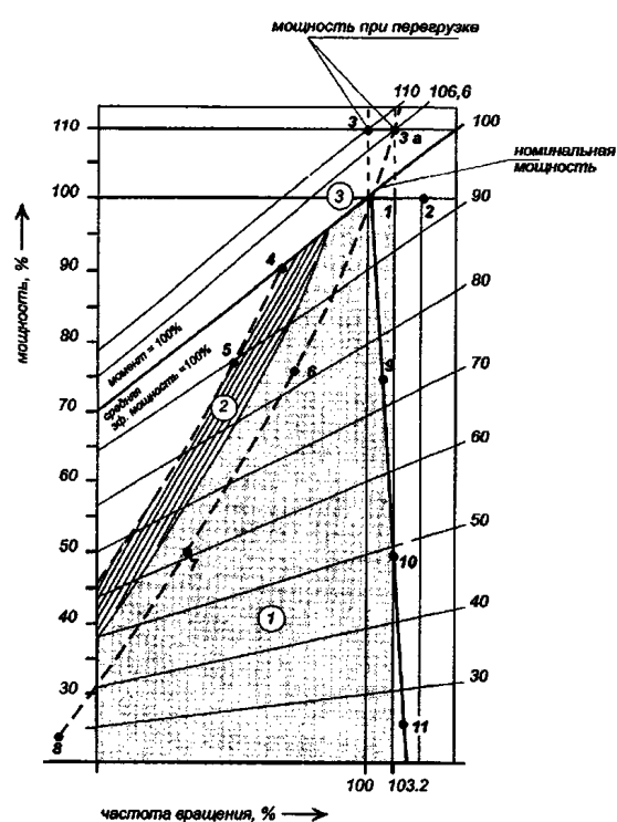
Рис. 8.5 Диаграмма режимов:
