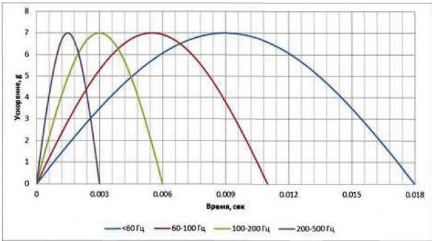
Рис. 2.5.2 Ударные импульсы при испытаниях на ударопрочность
