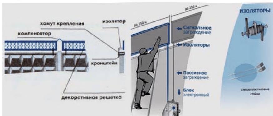
Рисунок 2.2 – Установка ЧЭ емкостного СО
