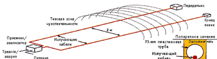
Рисунок 2.17 – Структурная схема ЛВВ-извещателя
