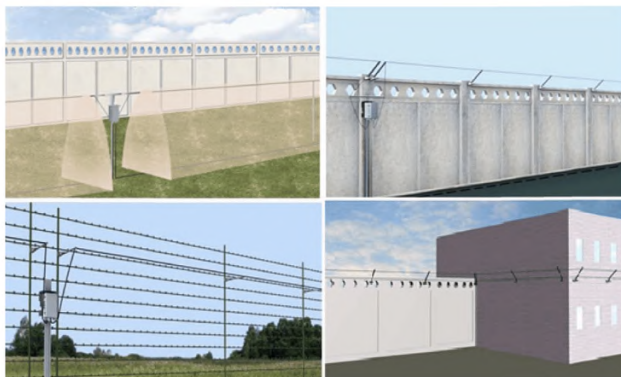
Рисунок 2.14 – Варианты установки проводноволнового извещателя
