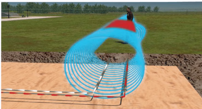
Рисунок 2.18 – Типовая ЗО при установке ЧЭ в грунт
