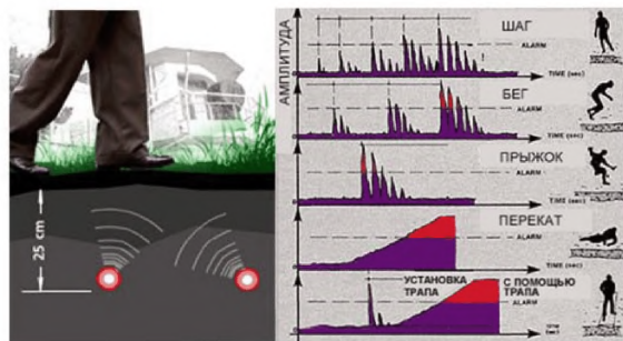
Рисунок 2.31 – Воздействие человека на ЧЗ и виды сигнала при пересечении ЗО
