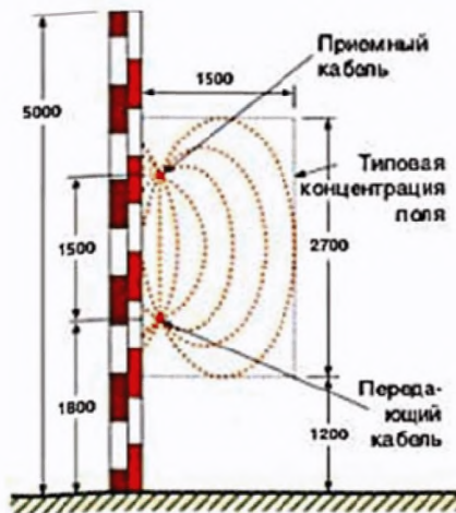
Рисунок 2.19 – Типовая 30 при установке ЧЭ на стене
