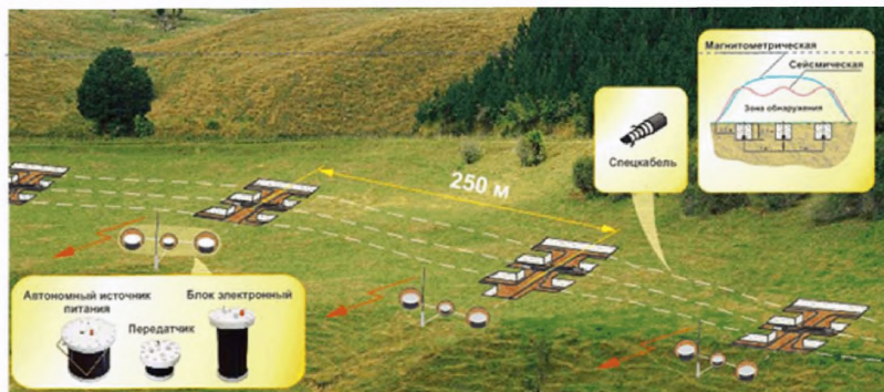
Рисунок 2.26 – Сейсмоманометрическое радиоканальное СО «Дуплет-Р»
