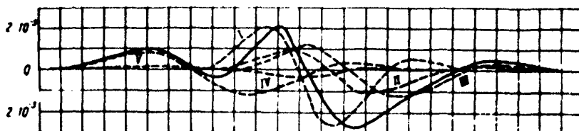
Рис. 19. Графики к примеру расчета сдвижений и деформаций земной поверхности. I, II, III, IV - соответственно от лав № I, II, III и IV V - мульда активизации; VI - суммарные сдвигения и деформации
