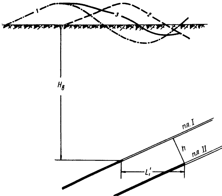
Рис.5. Схема к определению расстояния L'_i при заданном положении нижней границы очистной выработки в верхнем пласте: 1-горизонтальные деформации от пласта I; 2-горизонтальные деформации от пласта II; 3-суммарные горизонтальные деформации от пластов I и II
