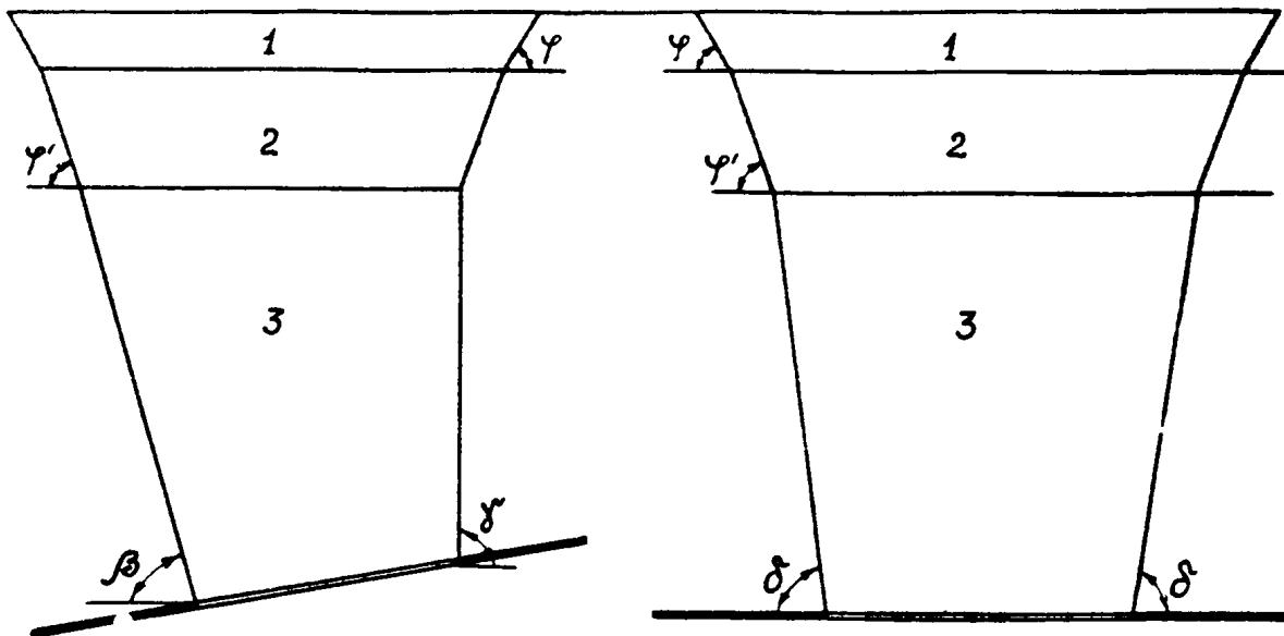
Рис.3. Определение границ зоны вредного влияния на земной поверхности: 1 - наносы; 2 - меловые отложения; 3 - каменноугольные породы.
