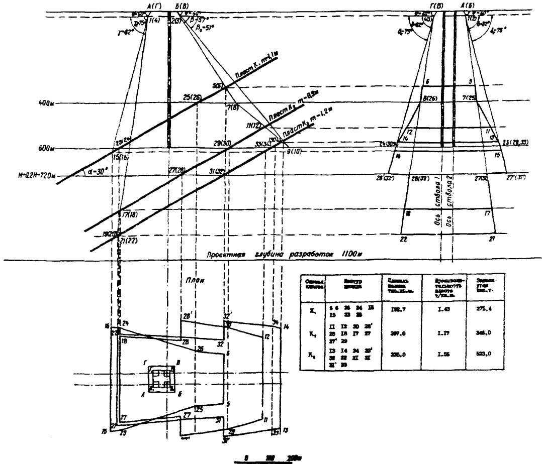
Рис.10. Пример построения предохранительных целиков в 3х пластах для охраны двух вертикальных шахтных стволов.
