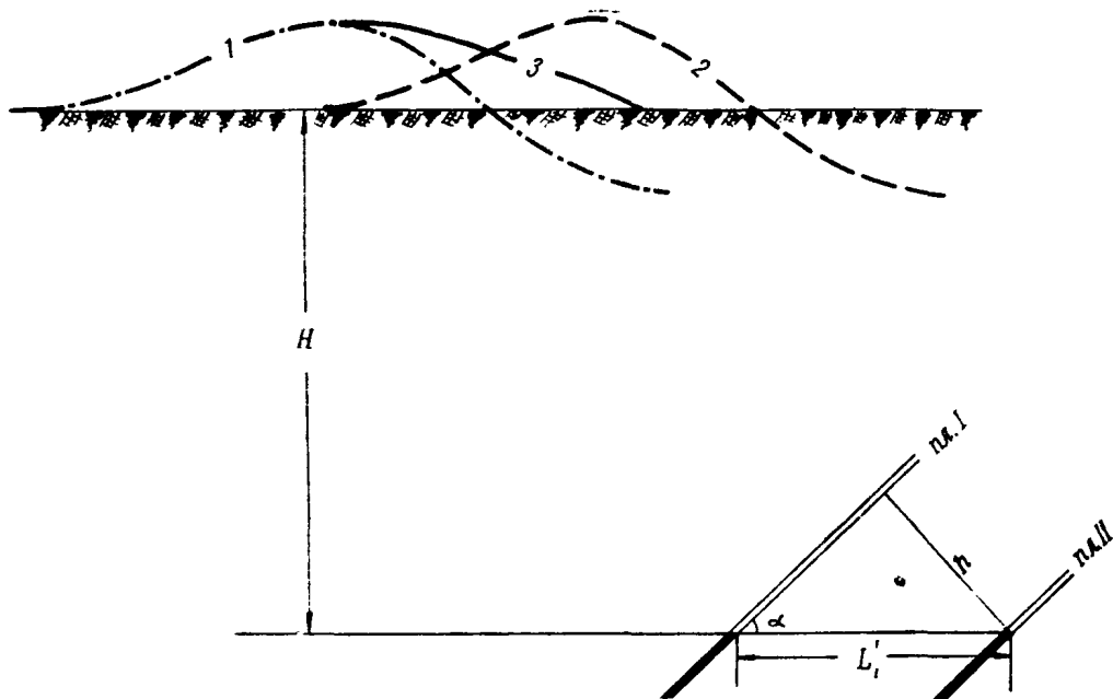
Рис.7. Схема к определению расстояний L'_i при заданной глубине горизонта отработки пластов: 1 - горизонтальные деформации от пласта I; 2 - горизонтальные деформации от пласта II; 3 - горизонтальные деформации от пластов I и II.
