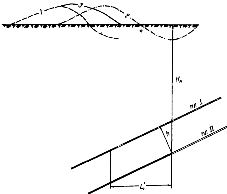
Рис.6. Схема к определению расстояния L' , при заданном положении нижней границы очистной выработки в нижнем пласте: 1 - горизонтальные деформации от пласта I; 2 - горизонтальные деформации от пласта II; 3 - суммарные горизонтальные деформации от пластов I и II.
