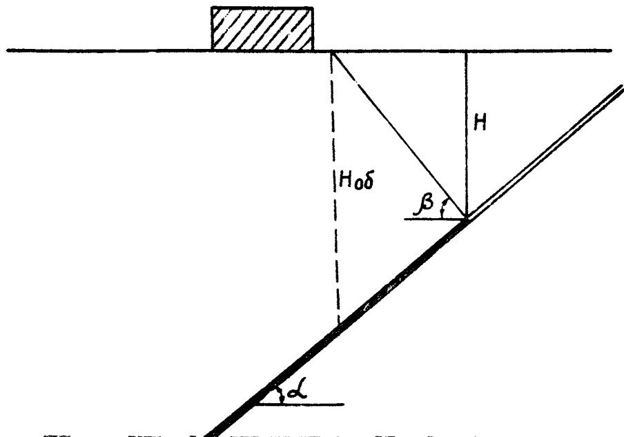
Рис.4. Определение глубины H , необходимой для получения угла \beta
