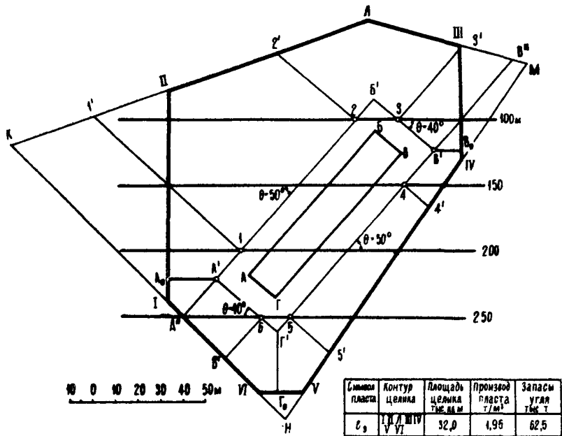
Рис.12. Пример построения предохранительного целика для охраны здания гаража
