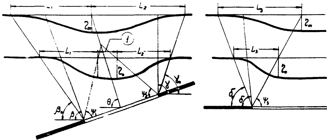
Рис.15. Исходные параметры процесса сдвигания: I-участок плоского дна мульдн.
