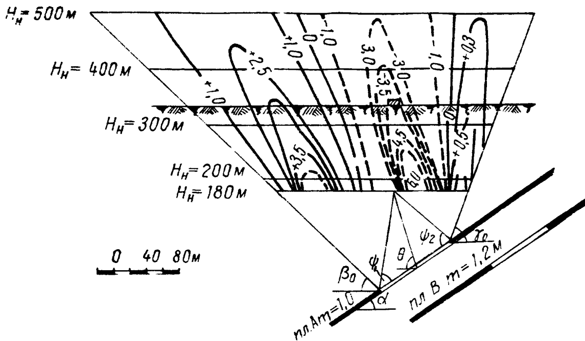
Рис.24. Схема к выбору местоположения очистной выработки в пласте А с помощью номограммы.
