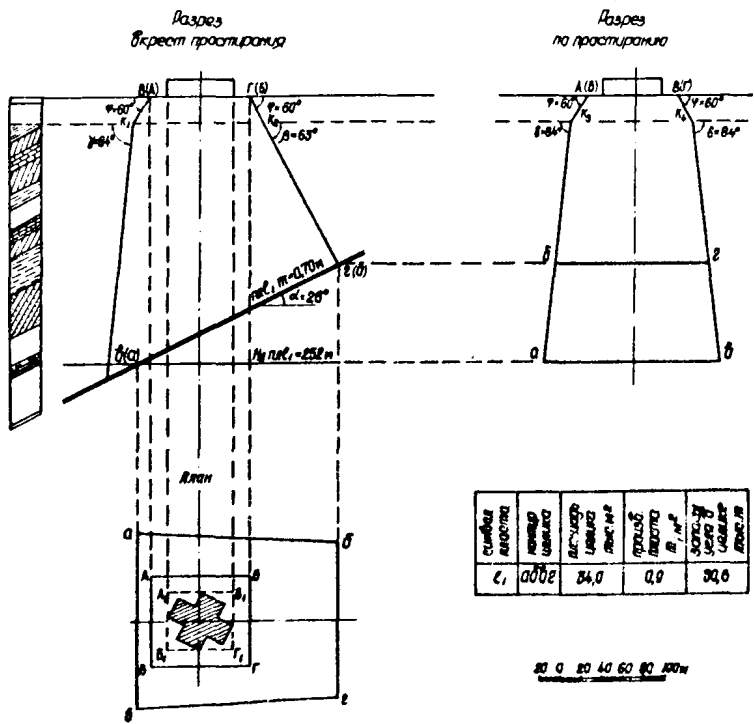
Рис.9. Пример построения предохранительного целина для охраны здания.
