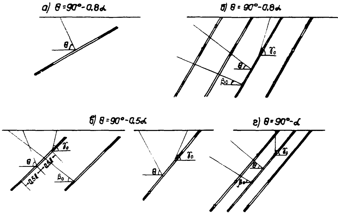
Рис.16. Схемы к понятию подрабстанности толщи горных пород.
