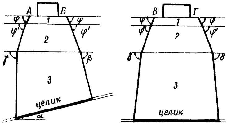
Рис.8. Определение границ предохранительного целика:
