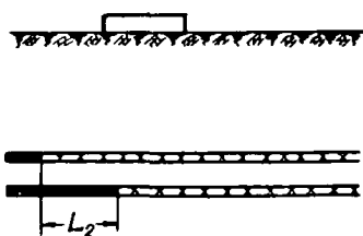
Рис. 29. Схема определения наилучшего, по условиям компенсации деформаций, расположения очистных выработок при одновременной разработке свиты угольных пластов по простраанию
