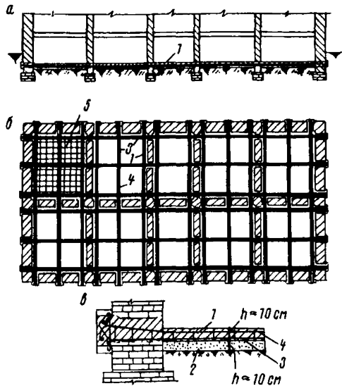
Рис. 41. Схема железобетонной плиты по грунту а - разрез, б - план, в - схема анкернения основных рабочих стержней плиты в наружной стене. 1- железобетонная плита h = 10-12 см, 2- песочная подушка, 3 и 4- верхняя и нижняя рабочая арматура плиты, 5- верхняя и нижняя арматурная сетка.
