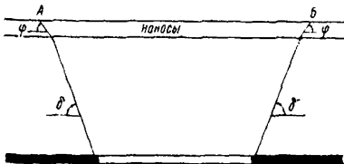
Рис. I. Определение границ зоны опасного влияния подземных разработок.
