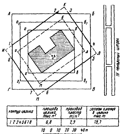
Рис. 4. Пример построения предохранительного целика для охраны здания школы.
