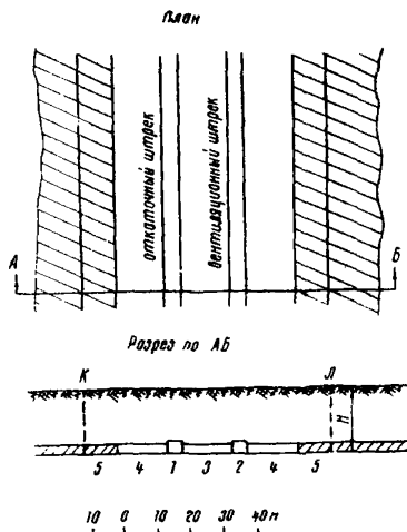
Рис. 3. Определение ширины участка над главными и панельными штреками, не подлежащего застройке.
