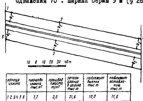
Рис.5. Пример построения предохранительного целика для охраны трубопровода.
