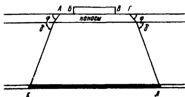
Рис.2. Определение границ предохранительного целика.
