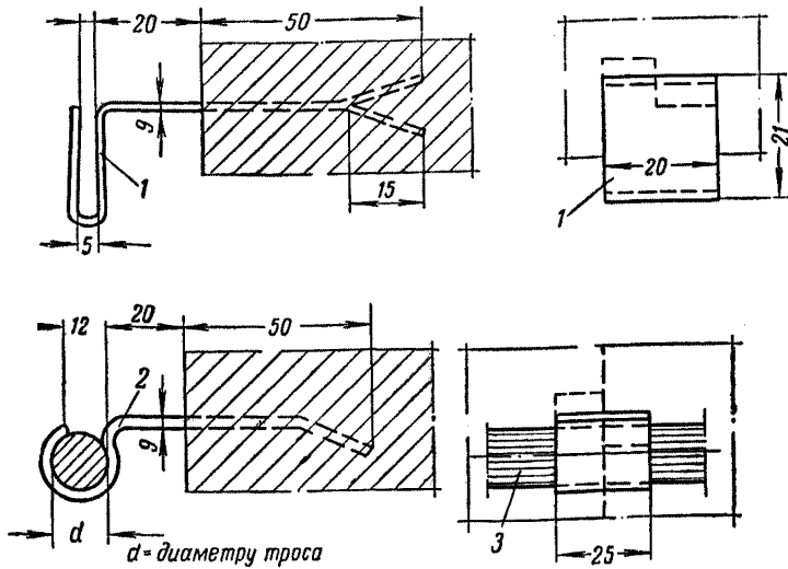
Рис. 17. Крепление заземляющей магистрали в камере с бетонной крепью: 1 — зажим для крепления плоских шин; 2 — зажим для троса; 3 — трос
