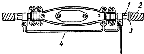
Рис. 6. Заземление соединительной муфты:
