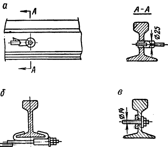
Рис. 23. Присоединение заземляющего проводника к рельсу:
