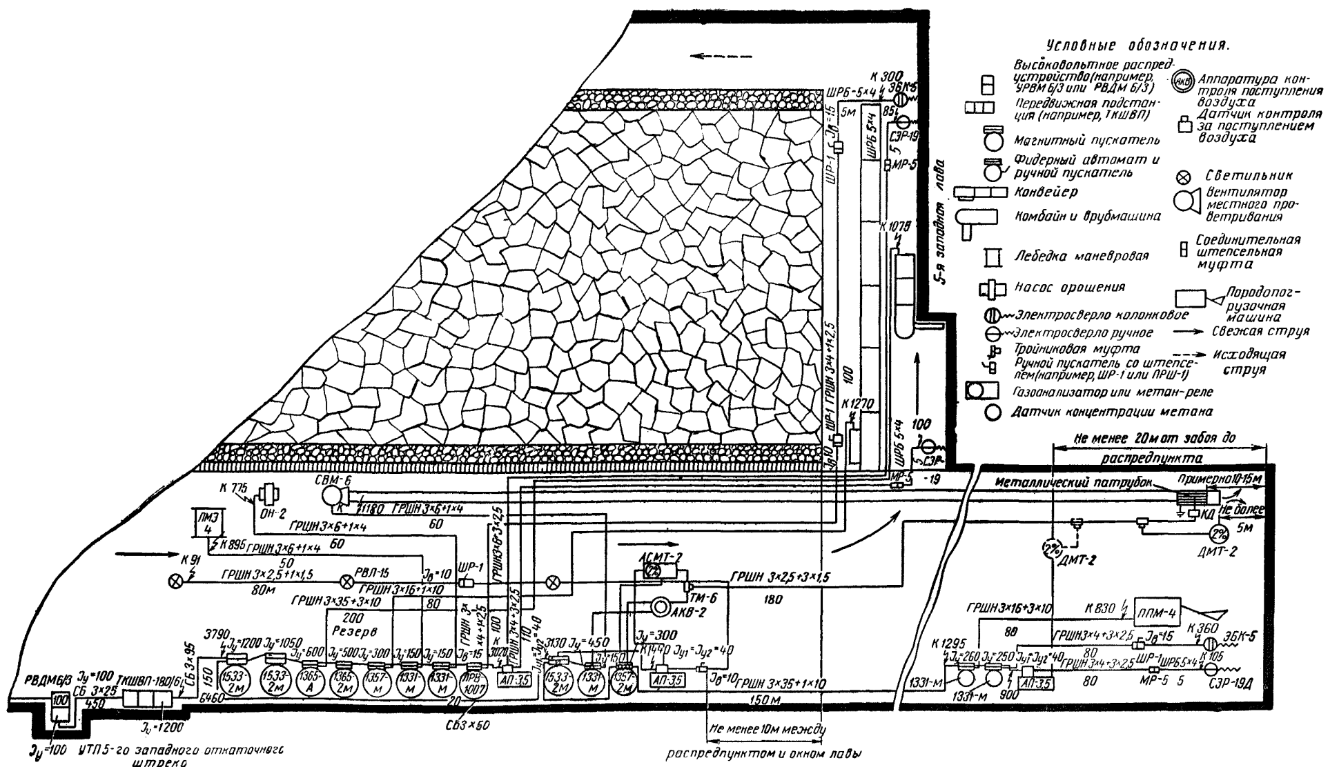
Рис. 3. Схема электроснабжения участка
