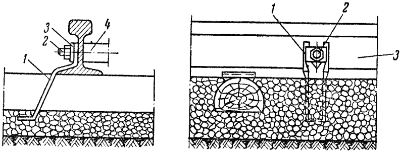
Рис. 20. Соединение заземляющего проводника с шейкой рельса с помощью хомута: 1 — заземляющий проводник 25 \times 5 мм; 2 — болт; 3 — шайба; 4 — между- рельсовая стяжка
