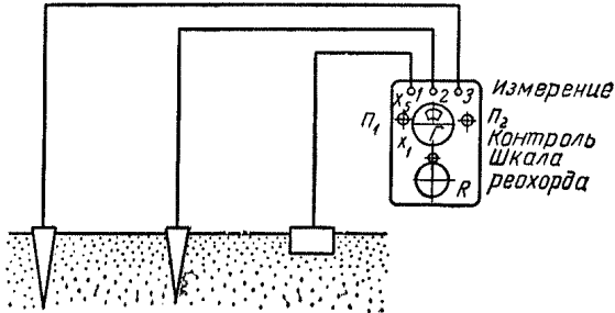
Рис. 27. Схема присоединения прибора М1103 при измерении сопротивления заземлителя
