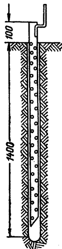
Рис. 3. Устройство заземления с помощью трубы
