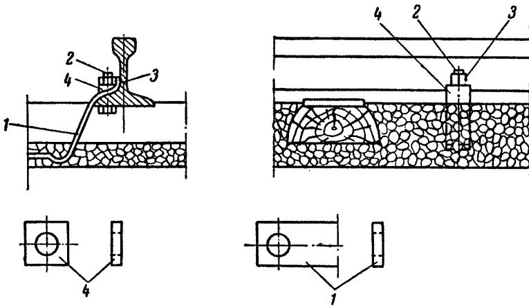
Рис. 21. Соединение заземляющего проводника с подошвой рельса (болтовое соединение): 1 — заземляющий проводник 25 \times 5 мм; 2 — болт; 3 — гайка; 4 — шайба
