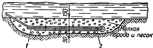
Рис. 2. Расположение заземлителя в сточной канаве:
