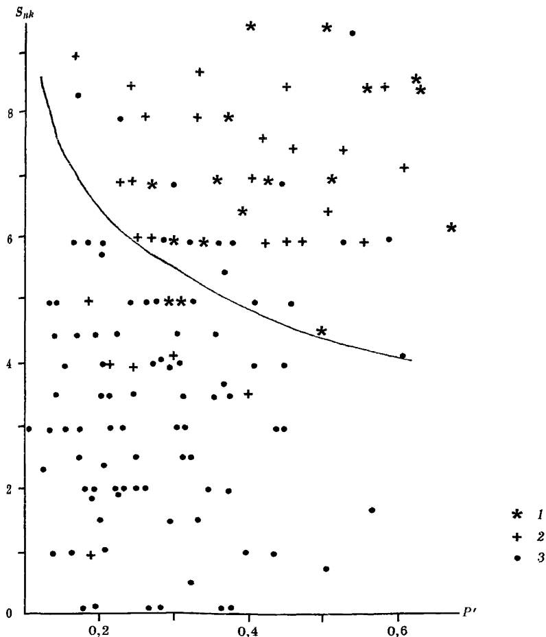
Рис. 7.13. Статистическая схема прогноза ЭВУЗВ по методу графической регрессии. 1 — P \geq 0,5 , 2 — 0,5 > P \geq 0,4 , 3 — P < 0,4 .
