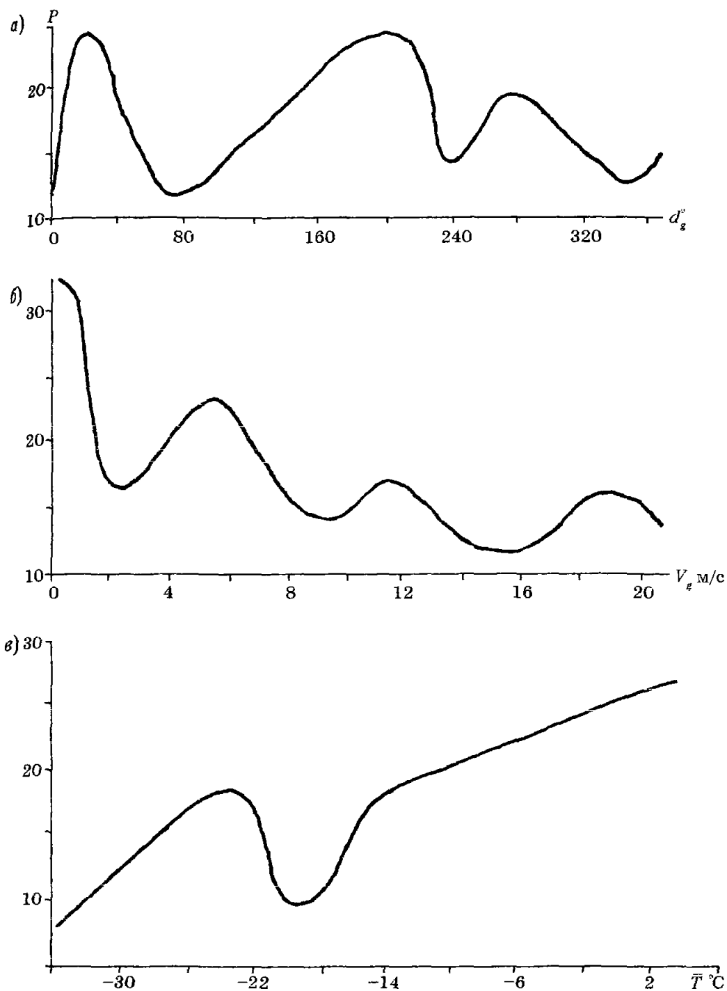
Рис. 9.1. Зависимость параметра P от предсказанных на 3 сут значений направления d_g (а) и скорости геострофического ветра V_g (б) и средней температуры воздуха \bar{T} в слое OT_{500/1000} (в).
