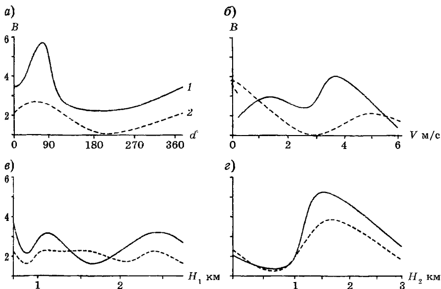
Рис. 8.1. Зависимость нормированной концентрации сероуглерода B на стационарных постах г. Красноярска от направления (а) и скорости (б) ветра, мощности приземной инверсии (в) и высоты нижней границы приподнятой инверсии (г). 1 — данные поста № 7, центр города; 2 — данные поста № 1, окраина города.
