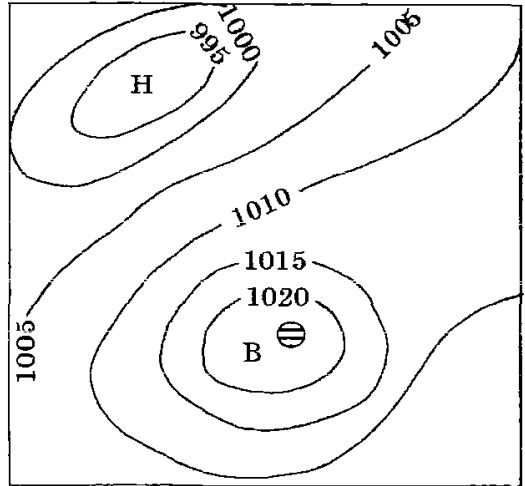
Рис. 7.1. Стационарный антициклон. Здесь и далее: заштрихованный круг — расположение города.
