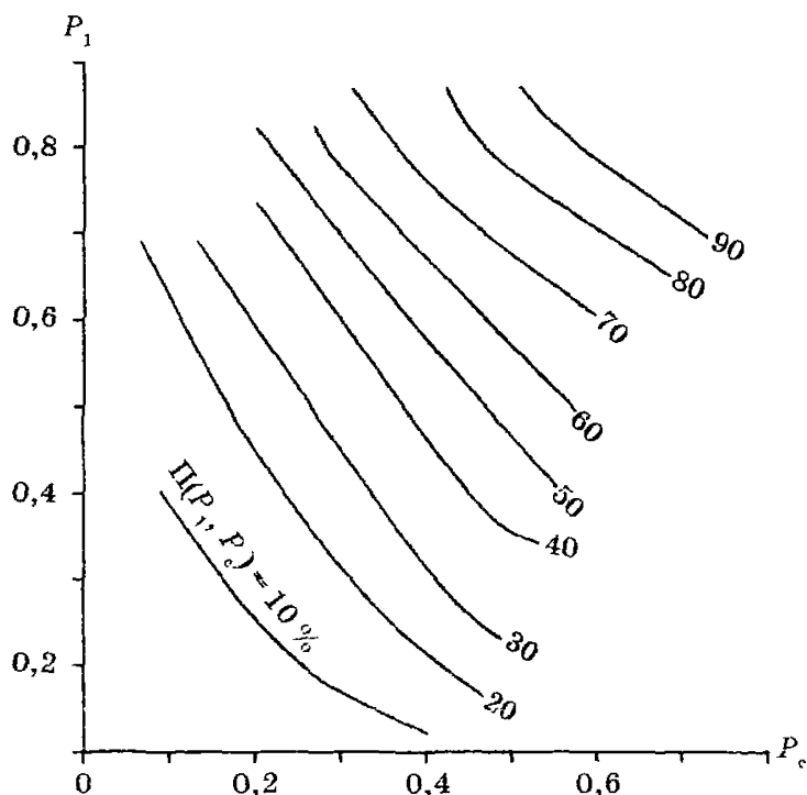
рис. 8.3. Предварительный график зависимости повторяемости \Pi повышенных значений V от параметров P_1 и P_c .
