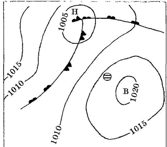
Рис. 7.4. Антициклон в теплой воздуш- ной массе.
