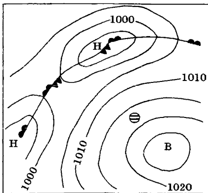
Рис. 7.8. Северо-западная периферия антициклона в сочетании с циклоничностью западнее и северо-западнее без распространения на район данного города.
