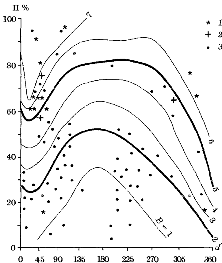
Рис. 8.4. Окончательный прогностический график. 1 — V > 5 , 2 — V = 4 \dots 5 , 3 — V < 4 . Изолинии значений V = 2 и V = 5 являются границами между 1-й и 2-й, а также между 2-й и 3-й группами оценок загрязнения воздуха.
