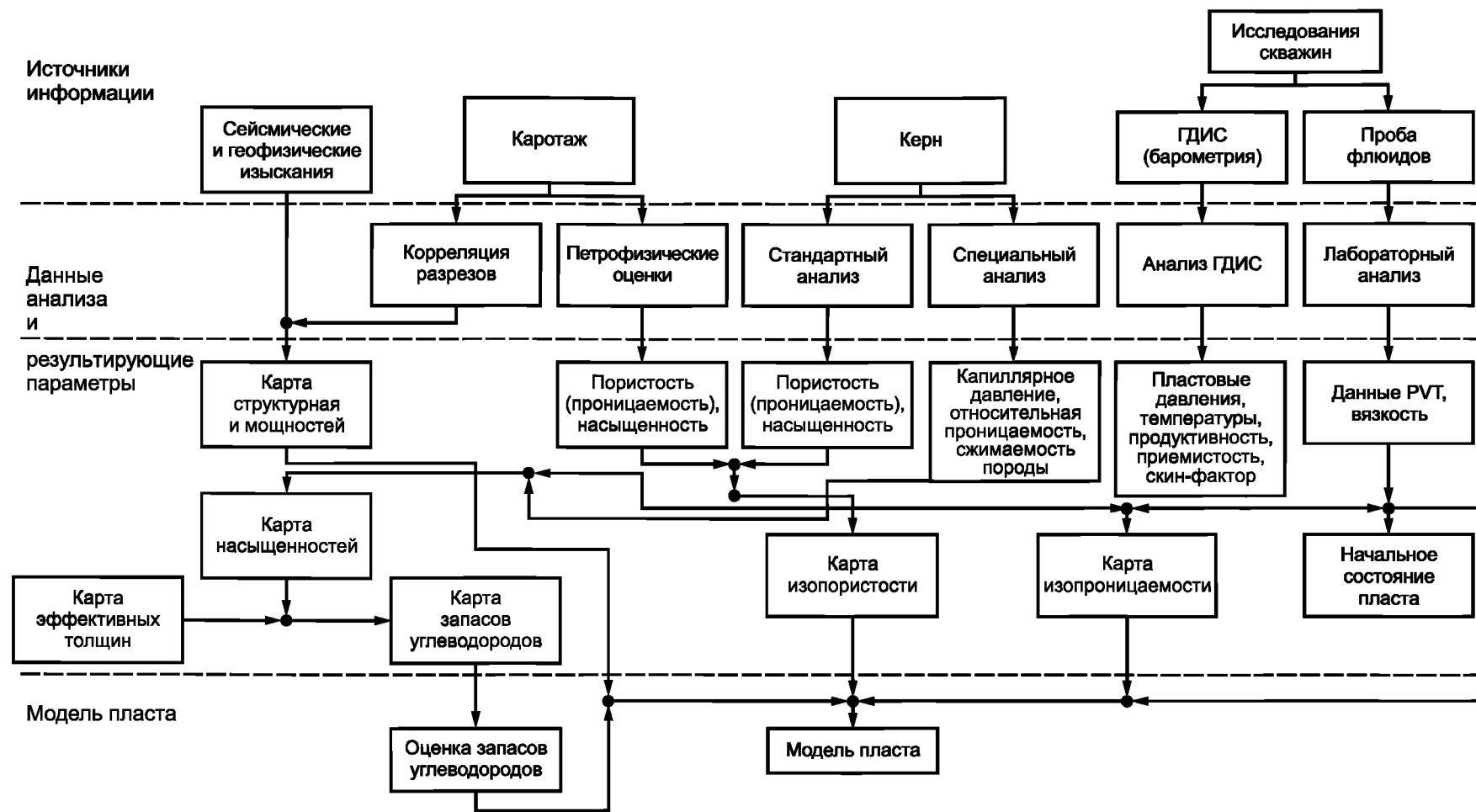
Рисунок 1 — Источники геолого-технологической информации о параметрах пласта и их использование
