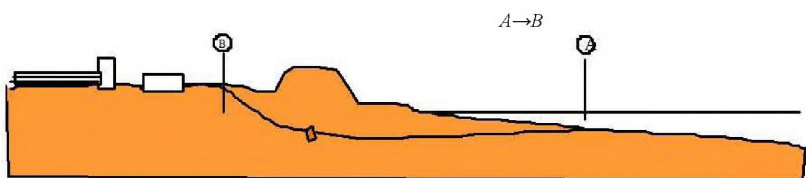
3. ННБ с суши с выходом в море
