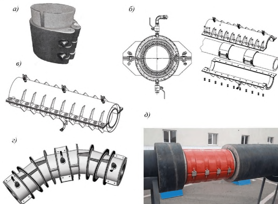
Рис. 12.3-2 Устройства для ремонта подводных трубопроводов, одобренные РС
