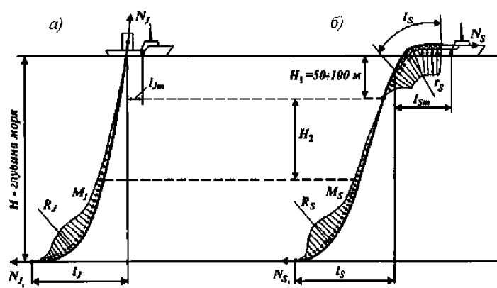
Рис. 7.1-3 Эпюры изгибающих моментов при укладке различными способами [1]: а — J -метод укладки; б — S -метод укладки
