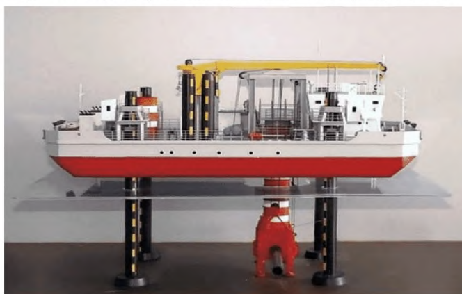
Рис. 12.3-3 Специализированное плавучее ремонтное средство СПРС-К (проект 91030)
