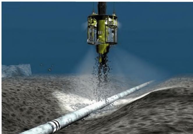
Рис. 12.1-3 Подбивка трубопровода на глубоководном участке
