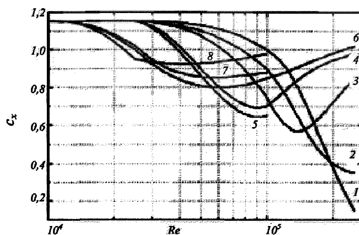
Рис. 4.3.1-3 График коэффициента c_x от числа Рейнольдса и относительной шероховатости поверхности трубы k : 1 — k = 0 ; 2 — k = 5,0 \cdot 10^{-4} ; 3 — k = 2,0 \cdot 10^{-4} ; 4 — k = 4,0 \cdot 10^{-3} ; 5 — k = 5,0 \cdot 10^{-3} ; 6 — k = 7,0 \cdot 10^{-3} ; 7 — k = 9,0 \cdot 10^{-3} ; 8 — k = 2,0 \cdot 10^{-2}
