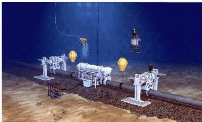
Рис. 12.2.1 Ремонтная система трубопровода Nord Stream с использованием гипербарической сварки Hyperbaric Welding System
