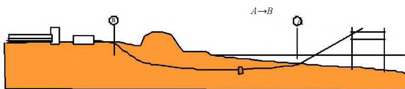
2. ННБ с буровой установки, установленной на морской буровой платформе
