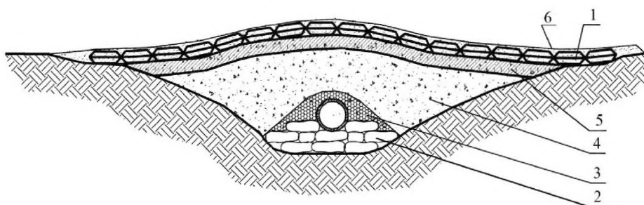
Рис. 12.1-2 Схема ремонта размыва с использованием гибких бетонных матов: 1 — элемент гибкого бетонного мата; 2 — мешки с песком или ЦПС; 3 — мягкий грунт (песок); 4 — насыпной грунт; 5 — щебень; 6 — песок
