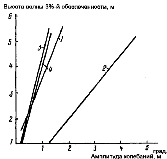
Рис. 7.3-1 Амплитуды качки на нерегулярном волнении 3-% обеспеченности ТУС SULEYMAN VEZIROV [2]:
