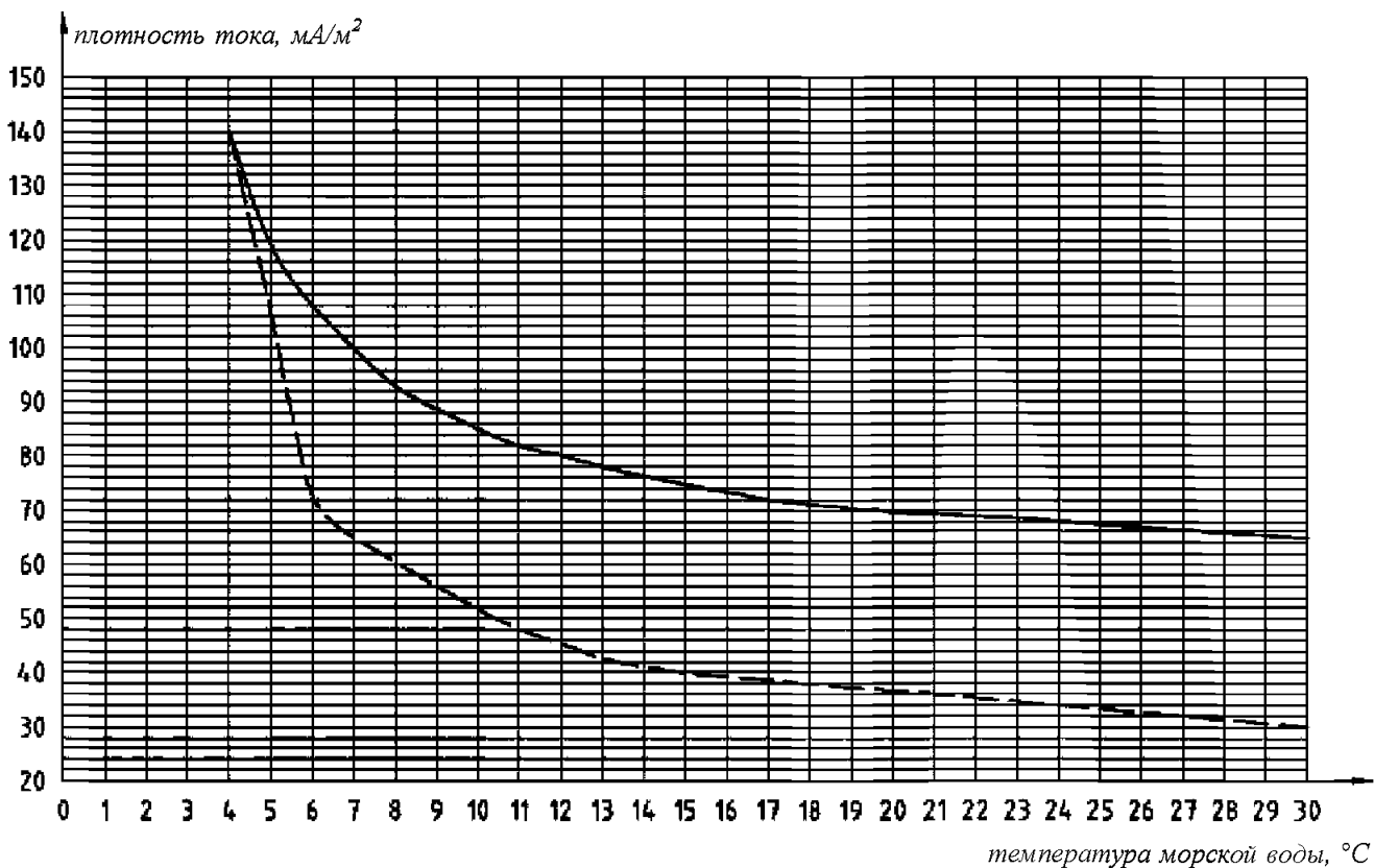
Рис. 8.4-3 Зависимость средней плотности тока от температуры воды
