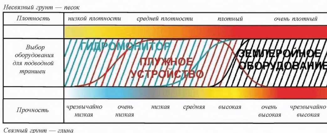
Рис. 10.2-3 Выбор технологии подготовки подводной траншеи [1]
