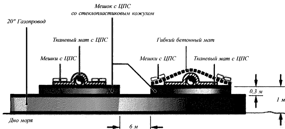
Рис. 11.2-2 Примеры конструктивных решений по пересечениям подводных трубопроводов [2]
