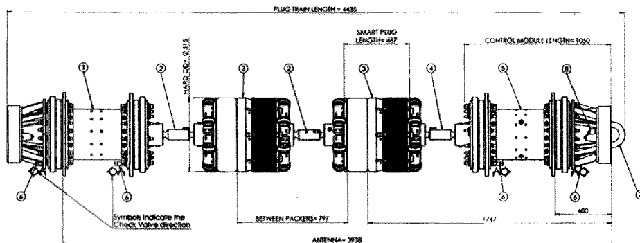
Рис. 12.3-4 Общий вид и компоновка затвора 2 × 24" типа SmartPlug:
