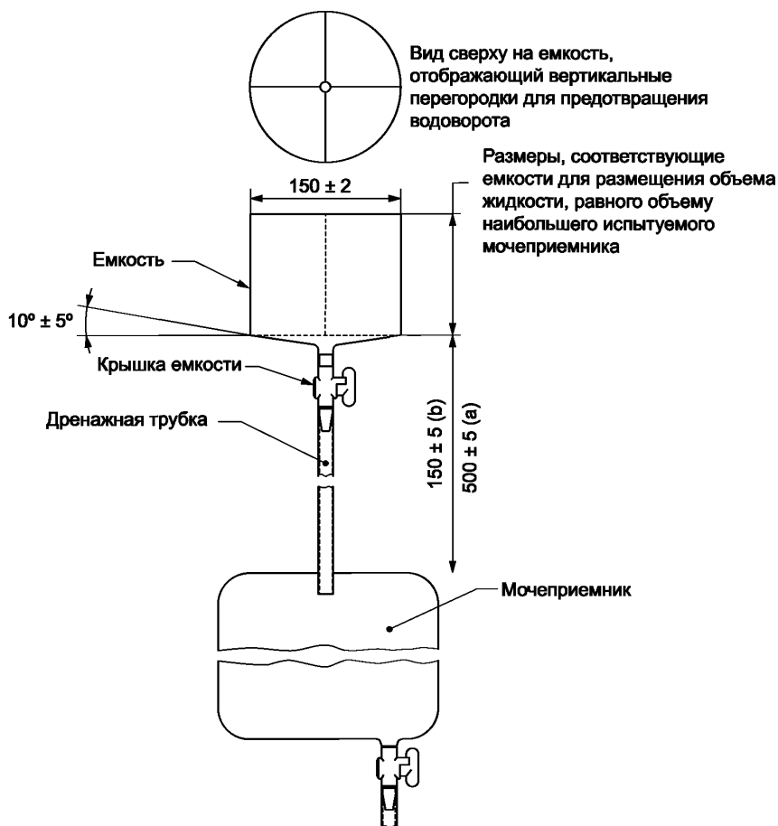
Рисунок 2 — Система заливки воды для испытания на отсутствие протекания (а) и измерения скорости наполнения (b)
