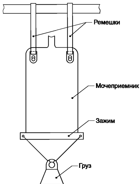
Рисунок 4 — Схема испытания на определение прочности системы крепления моче-приемников с пуговицами и петлями
