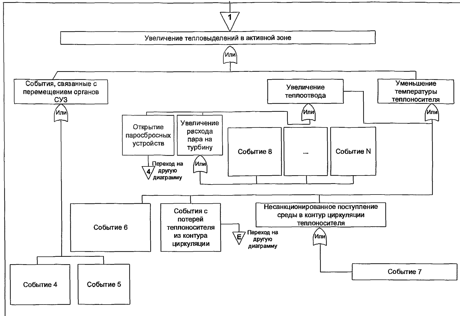
Рис. 2. Логическая диаграмма причин выхода РВ за установленные проектом границы (продолжение)
