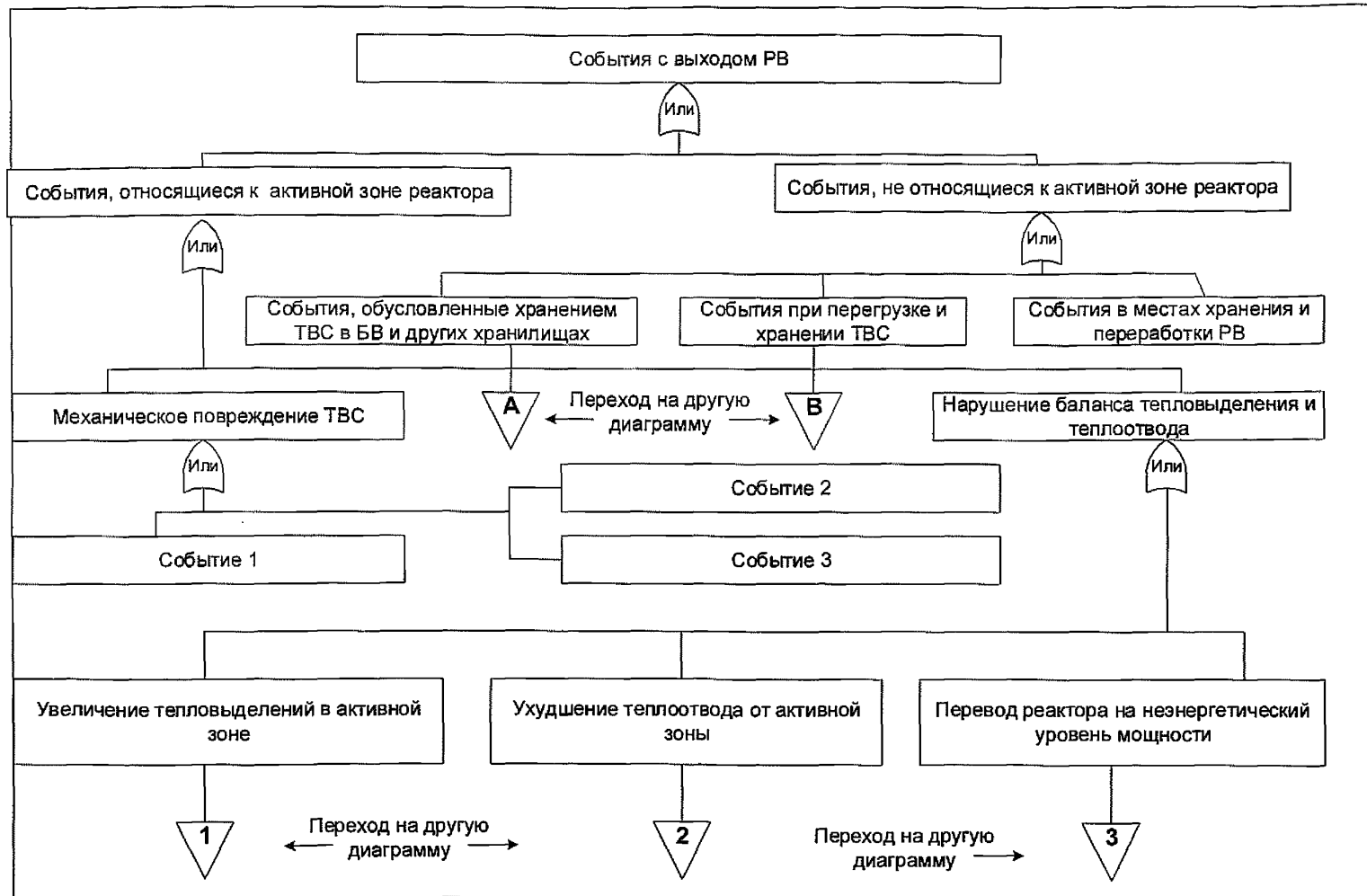
Рис. 1. Логическая диаграмма причин выхода РВ за установленные проектом границы
