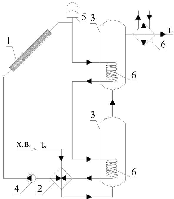
Рисунок Е.16 – Принципиальная схема двухконтурной гелиосистемы:
