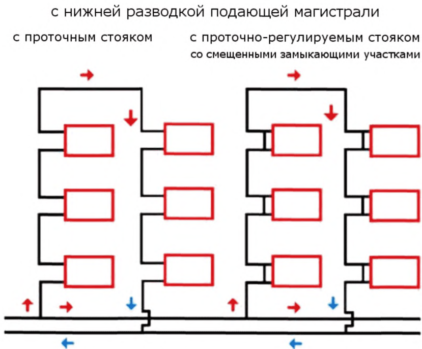
Рисунок Д.14 – Однотрубные вертикальные системы.
