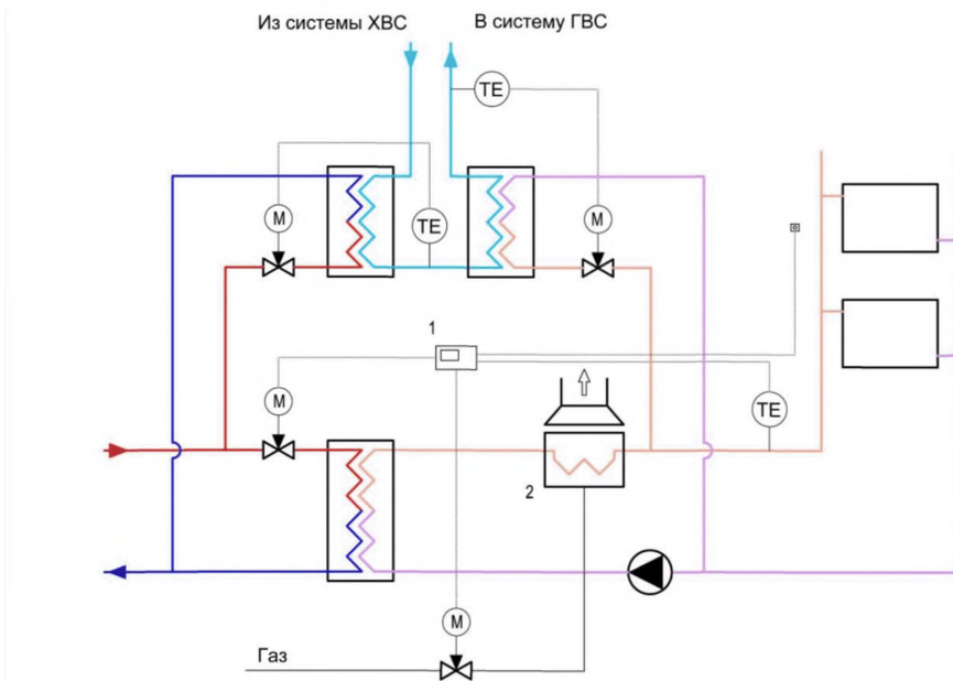
Рисунок Д.33 – Схема теплового пункта с пиковым газовым котлом.
