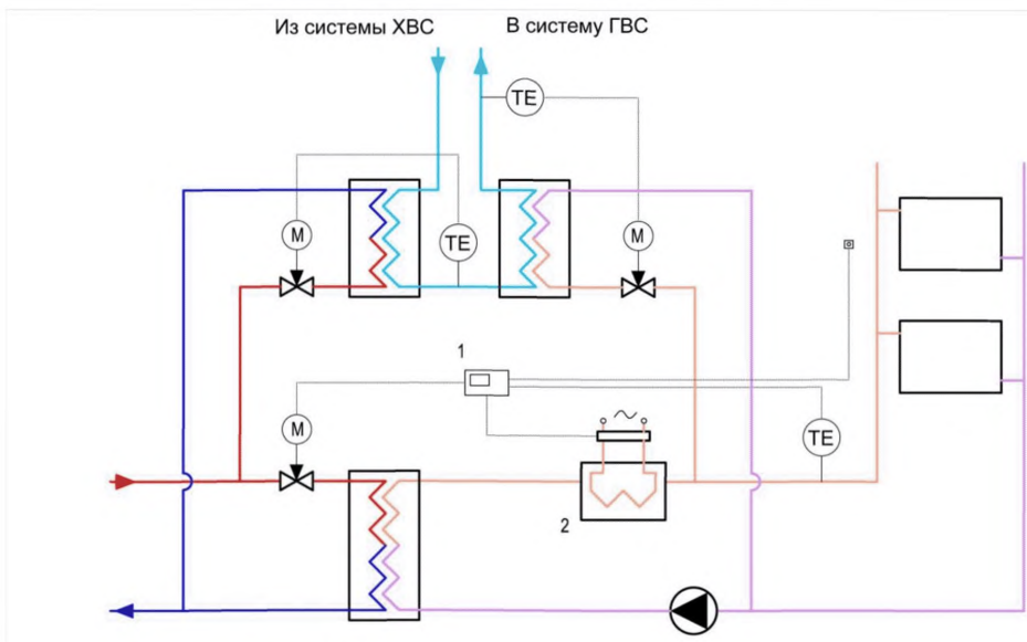
Рисунок Д.34 – Схема теплового пункта с электроподогревателем
