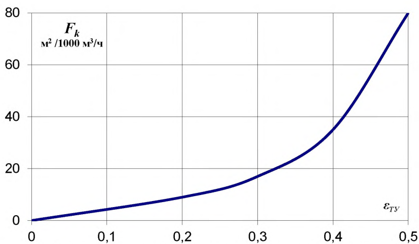
Рисунок Е.3 – Зависимость площади теплопередачи калориферов-теплоутилизаторов от степени утилизации \varepsilon_{TY}
