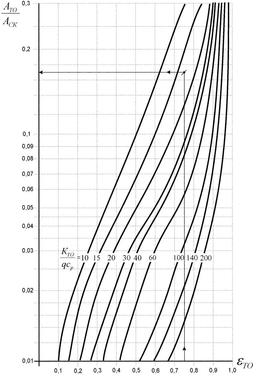
Рисунок Е.19 – График определения относительной площади теплообменника
