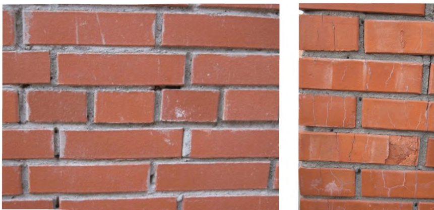
Рисунок А.2.1. Не полное заполнение горизонтальных и вертикальных растворных швов кладки (пустошовка)
