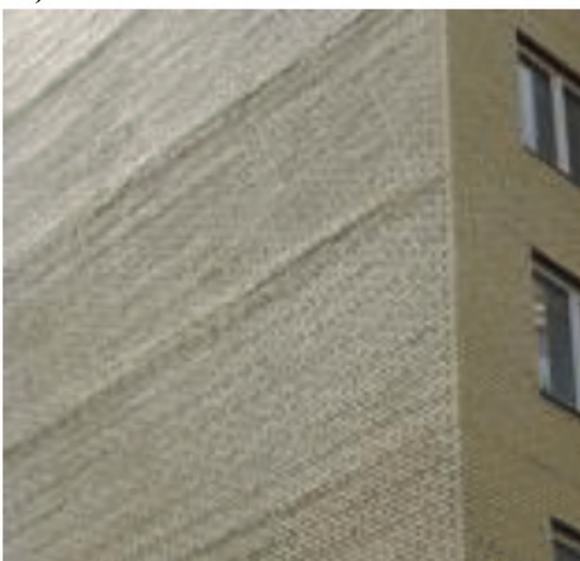
Рисунок А.1.2. Выпучивание облицовочного слоя из-за отсутствия горизонтальных деформационных швов, отсутствия либо недостаточного количества гибких связей:
