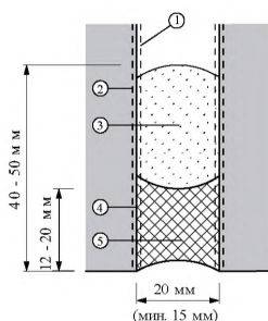
Рисунок 7.3 Уплотнение вертикальных (а) и горизонтальных (б) деформационных швов в облицовочном каменном слое
