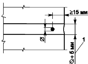
Рисунок 11.1 Защитный слой для арматуры, расположенной в горизонтальных швах
