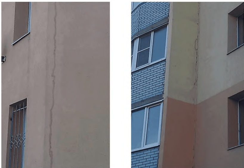
Рисунок Б.8. Дополнительное утепление фасада с оштукатуриванием тонким слоем без усиления армирования в угловых зонах здания
