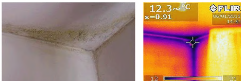
Рисунок А.1.17. Увлажнение внутри помещений из-за недостаточной теплоизоляции или протечек
