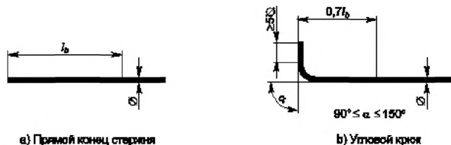
Рисунок 11.2. Анкеровка арматурных стержней в растворяемых швах
