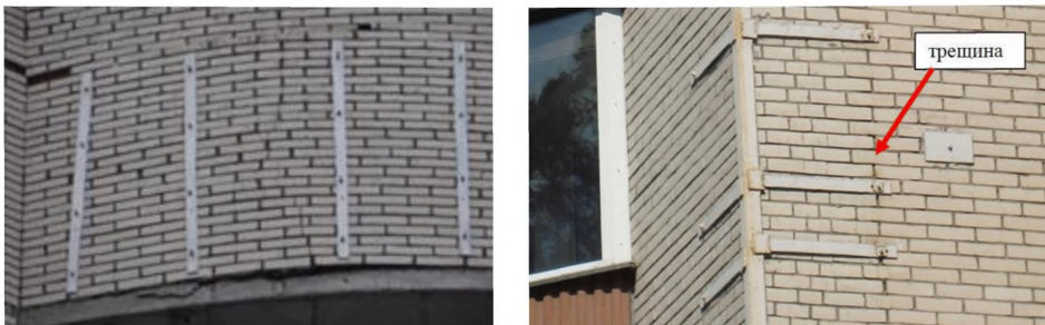
Рисунок Б.1. Укрепление участков облицовочного слоя с трещинами металлическими обоями
