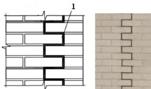
Рисунок 7.2. Устройство вертикального деформационного шва штрабой
