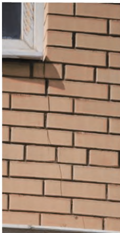
Рисунок А.1.6. Вертикальные и наклонные трещины на прямых участках стен в угловых зонах оконных проемов вследствие различных деформаций кладки в межоконных поясах и простенках и отсутствия ее армирования
