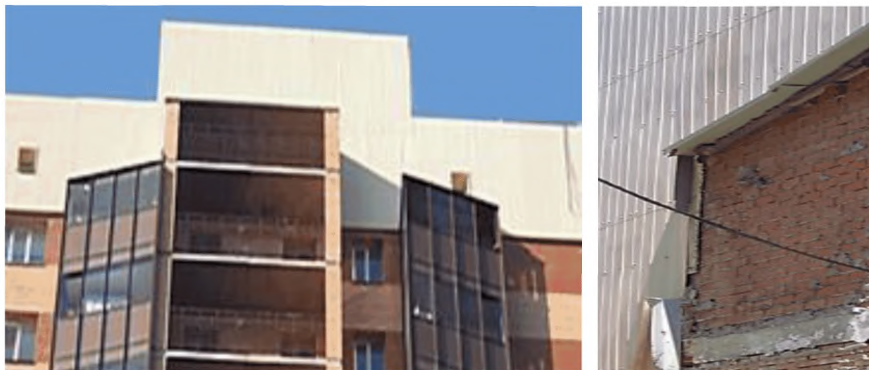
Рисунок Б.9. Защита поврежденного облицовочного каменного слоя сэндвич – панелями с низкой паропроницаемостью и высокой деформативностью при внешних температурных воздействиях
