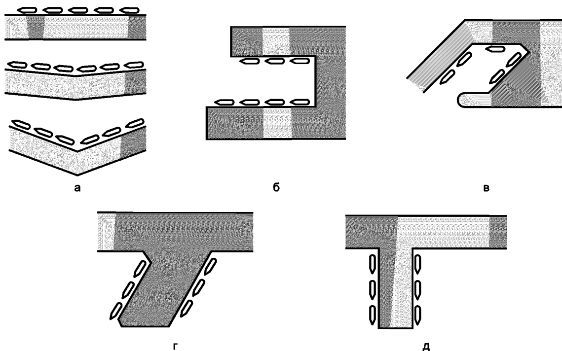
а — фронтальное; б, в — ковшовое; г, д — пирсовое
