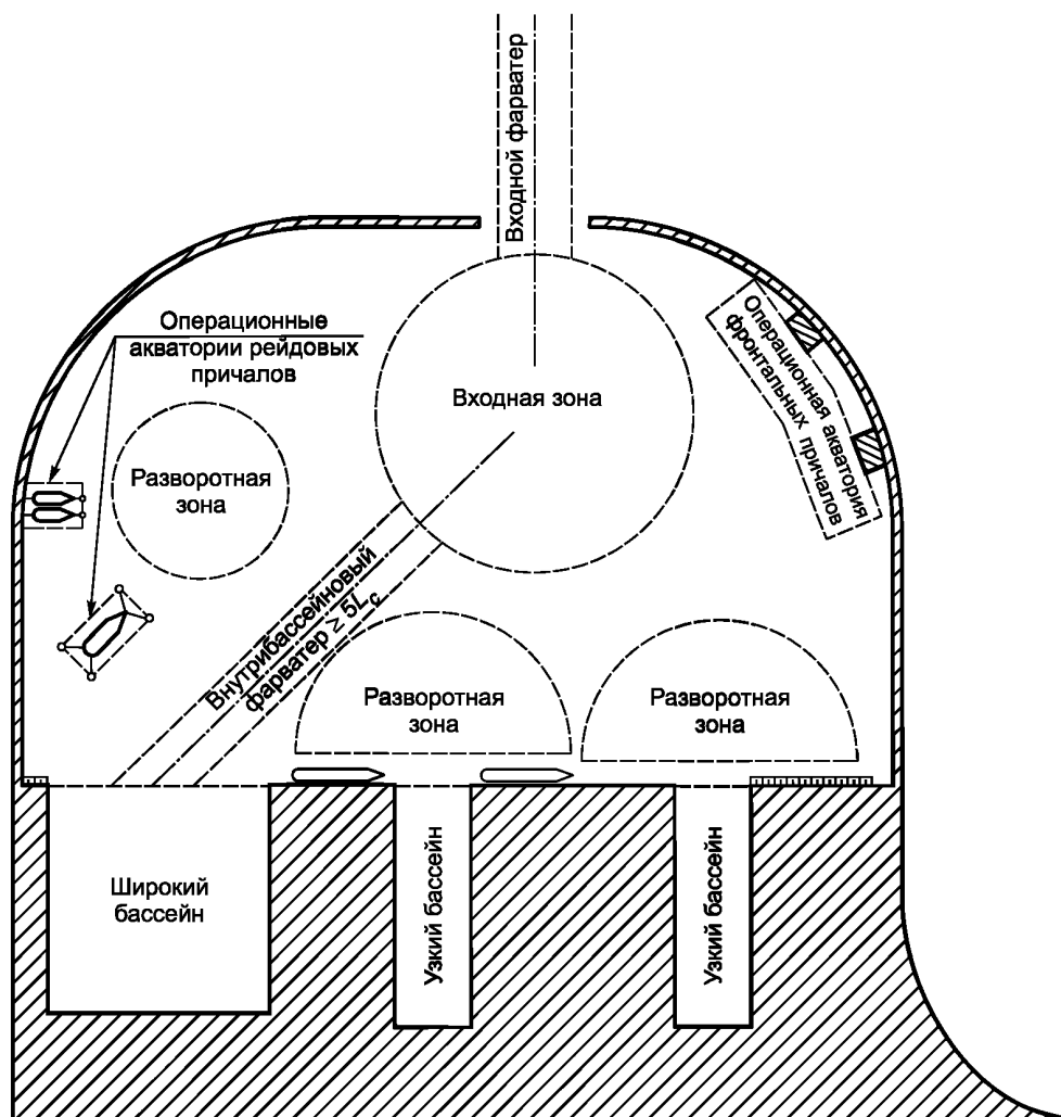
Рисунок А.2 — Схема расположения элементов внутренней акватории порта
