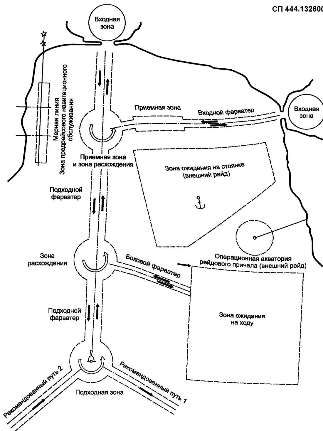
Рисунок А.1 — Схема расположения элементов внешней акватории порта и водных подходов
