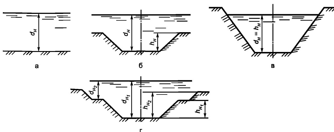
а) мелководье (фарватер); б) канал неполного профиля; в) канал полного профиля; г) канал переменного профиля
