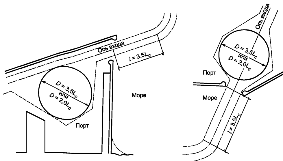
Рисунок 7.2 — Варианты организации входной зоны, а и б
