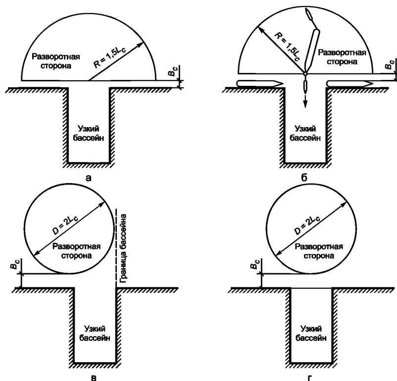
Рисунок 7.3 — Разворотная зона, непосредственно прилегающая к входу в узкий бассейн
