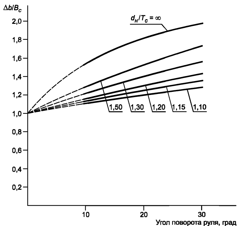
Рисунок В.2 — Определение уширения канала на повороте \Delta b
