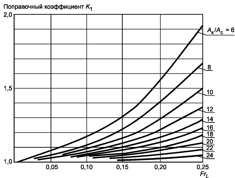
Рисунок 8.3 — Номограмма для определения поправочного коэффициента K_1 для канала неполного профиля по числу Фруда Fr_L и отношению площадей A_k/A_c
