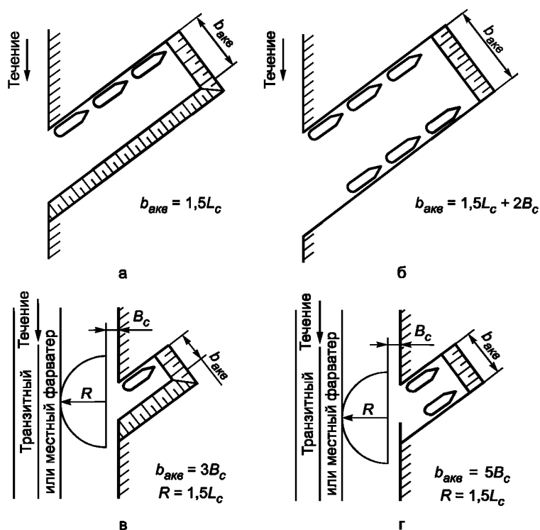
Рисунок 7.6 — Габариты бассейнов, расположенных на участках рек с морским режимом судоходства, а также бассейнов для судов портового и вспомогательного флота, двухвальных судов и судов с подруливающими устройствами дедвейтом до 10 тыс. т, расположенных на морских побережьях
