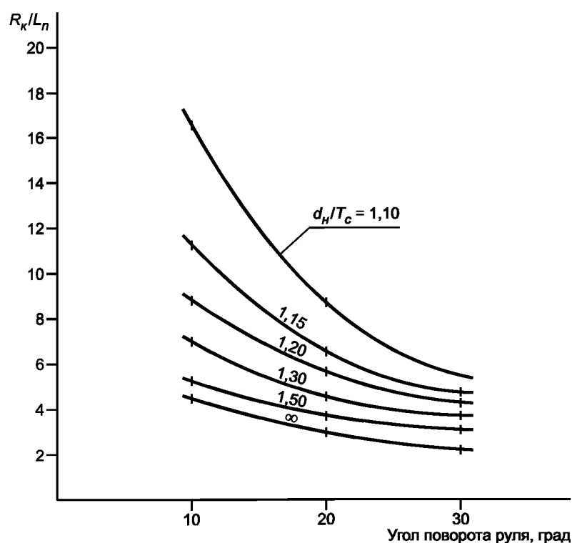
Рисунок В.1 — Определение радиуса закругления канала на повороте R_k
