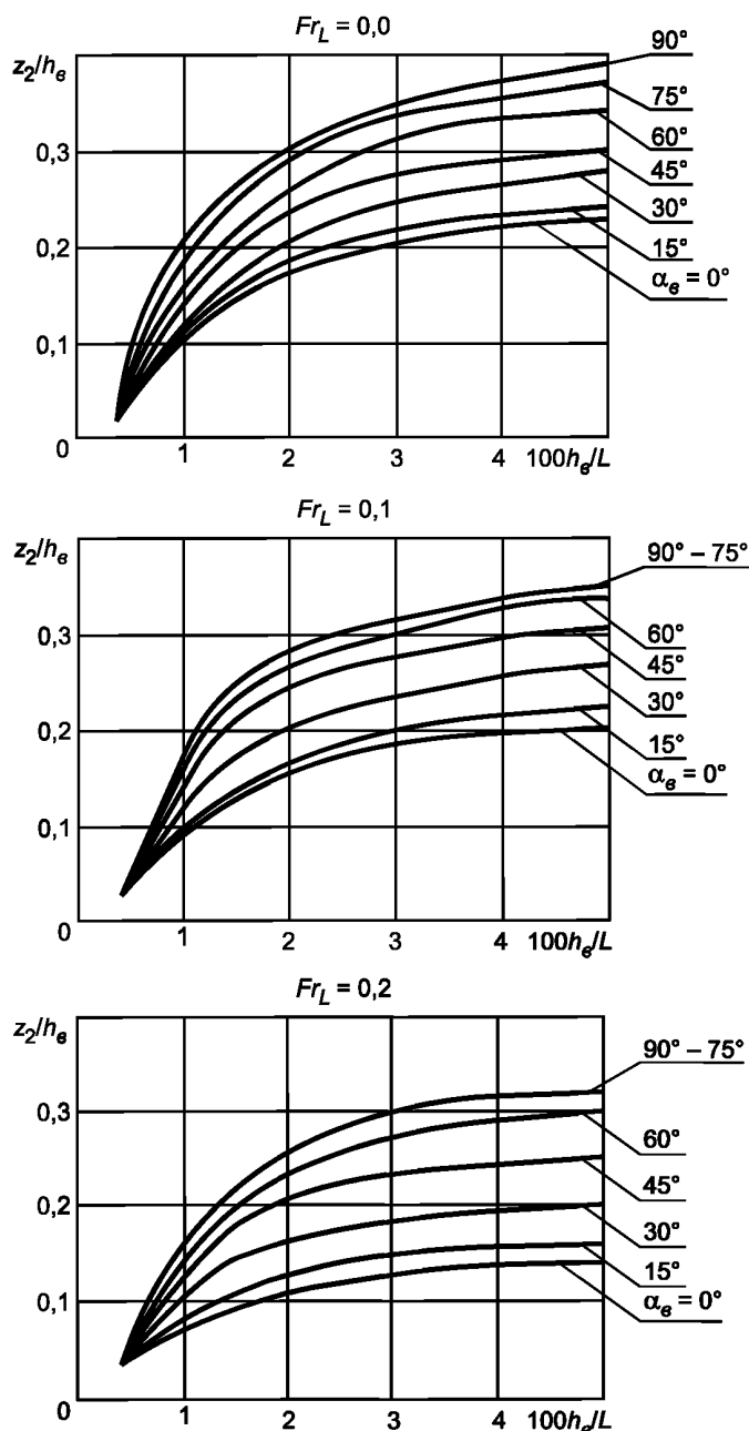
Рисунок 8.1 — Номограмма для определения отношения запаса от волновых воздействий к высоте волны z_2/h_B , при различных углах волнения \alpha_B и числах Фруда Fr_L
