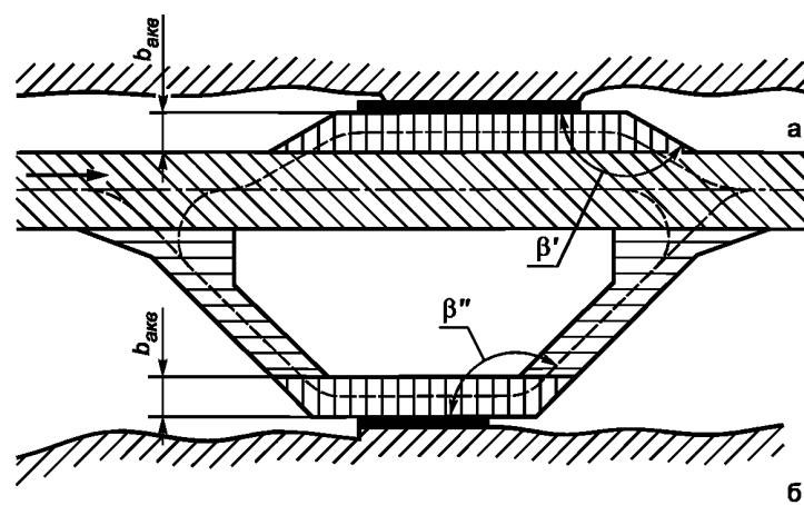
Рисунок 7.6 — Габариты бассейнов, расположенных на участках рек с морским режимом судоходства, а также бассейнов для судов портового и вспомогательного флота, двухвальных судов и судов с подруливающими устройствами дедвейтом до 10 тыс. т, расположенных на морских побережьях
