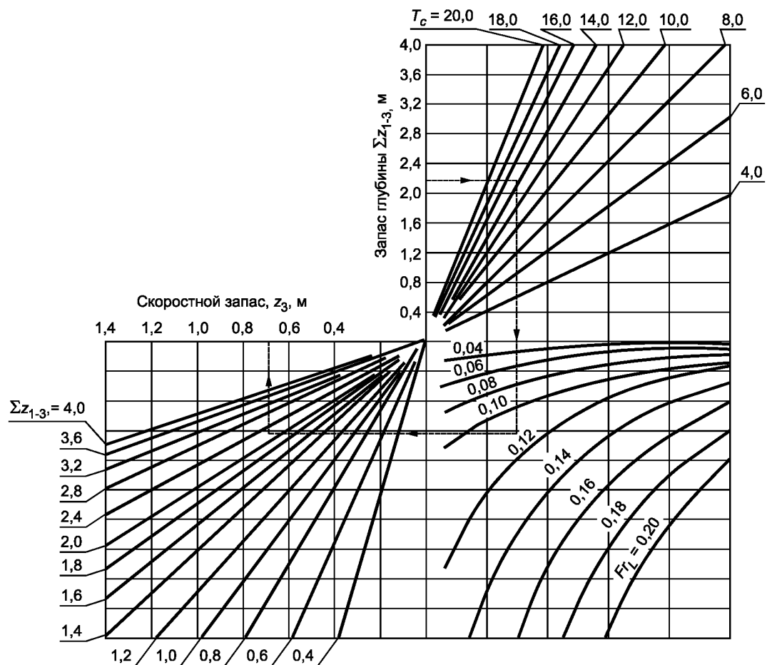
Рисунок 8.2 — Номограмма для определения скоростного запаса z_3 на мелководье по осадке судна T_c , числу Фруда Fr_L и суммарному запасу глубины \Sigma z_{1-3}
