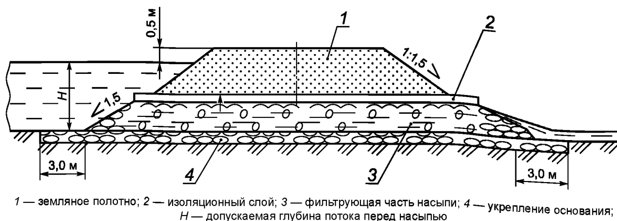
Рисунок А.3 — Напорные фильтрующие насыпи
