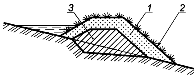
1 — дренарующий грунт; 2 — укрепление; 3 — водонепроницаемое ядро
