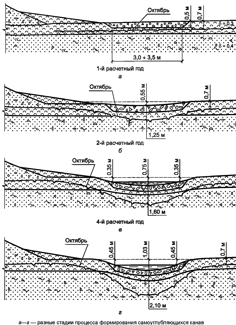
Рисунок В.7 — Водоотводная канава самоуглубляющегося типа, построенная на моховой мари с наличием близко залегающего к дневной поверхности подземного льда в долине реки
