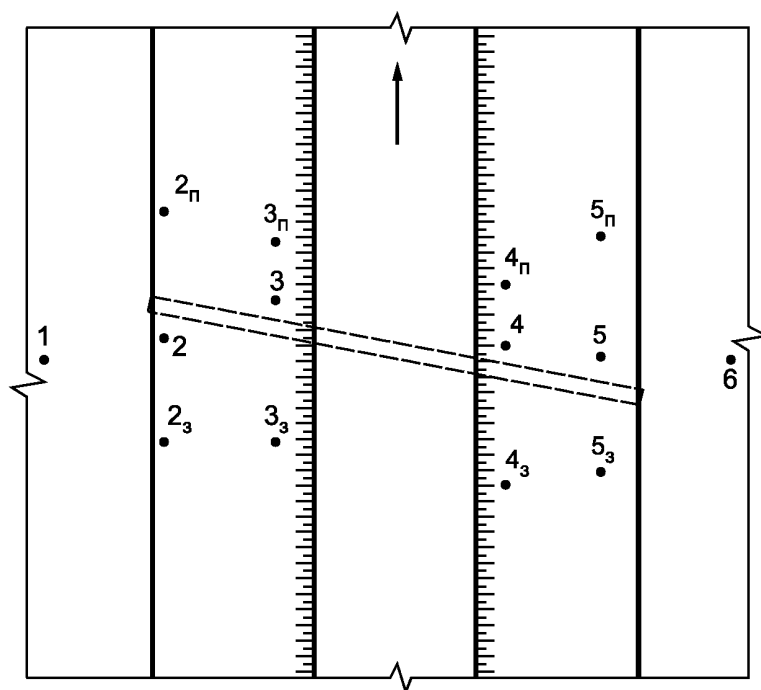
Рисунок Д.3 — Нумерация термоскважин в зоне водопропускной трубы
