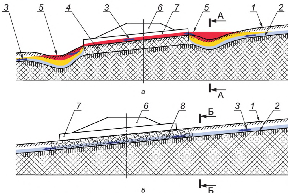
1 — естественная поверхность грунта; 2 — водопор; 3 — направление водного потока; 4 — массив уплотненного под насыпью грунта; 5 — верхний уровень воды; 6 — тело насыпи; 7 — водопропускная труба; 8 — крупнопористая скальная наброска под телом трубы
