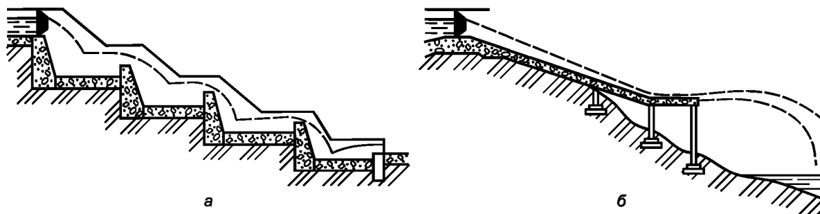
а — ступенчатый перепад; б — консольный перепад
