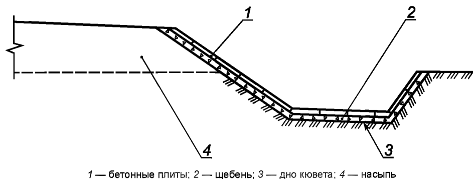
Рисунок А.6 — Кювет, укрепленный бетонными плитами
