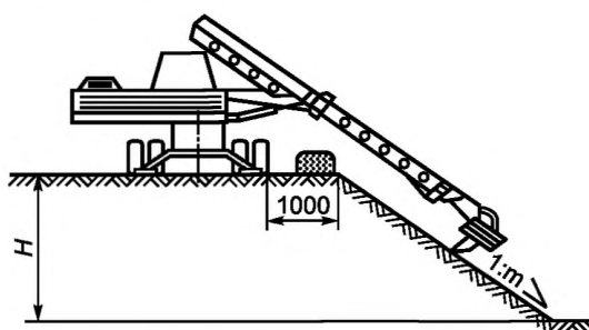
Рисунок А.13 — Планировка поверхности откоса ковшем
