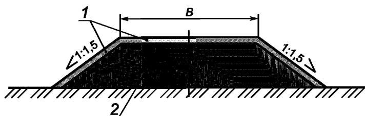
Рисунок А.8 — Поперечный профиль дамбы
