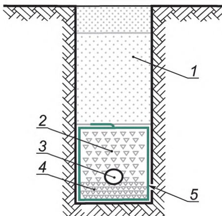
1 — песок; 2 — крупный щебень; 3 — труба; 4 — мелкий щебень; 5 — нетканый геотекстиль
