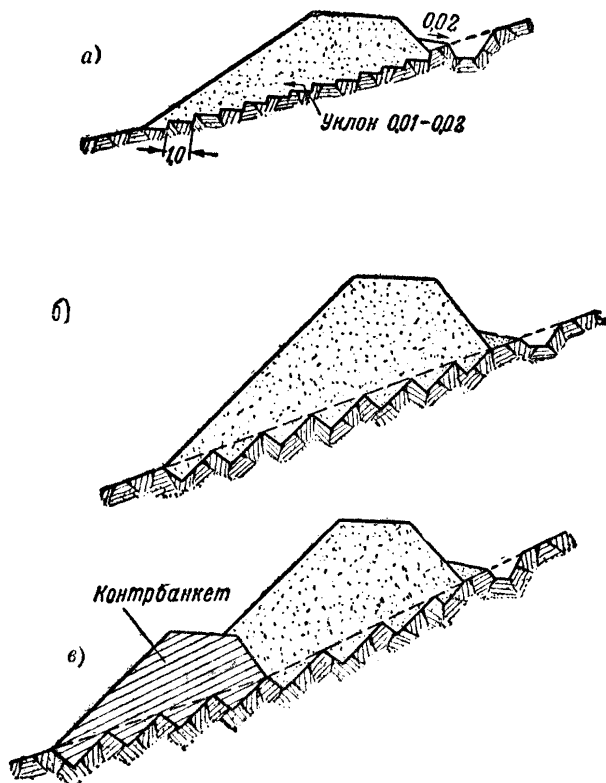
Фиг. 39. Схема устройства основания насыпей на косогорах
