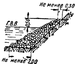
Фиг. 129. Обсыпка камнем
