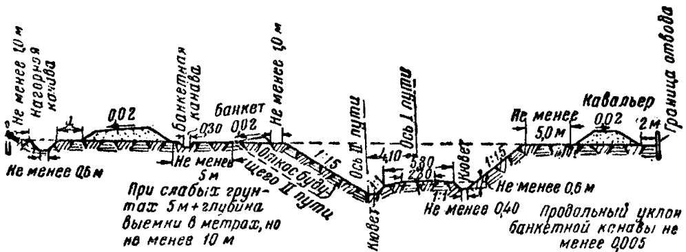
Фиг. 9. Выемка глубиной более 2 м с кавальерами
