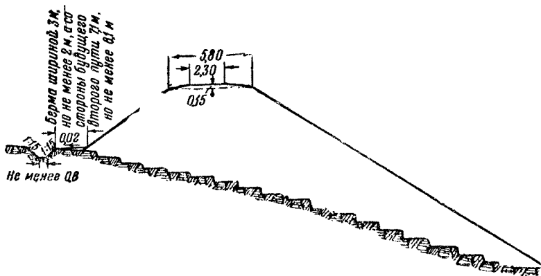
Фиг. 6. Насыпи на косогоре при крутизне более 1:5
