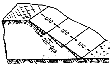
Фиг. 120. Схема устройства уступов на откосах для засыпки при укреплении корневой системой и с посевом
