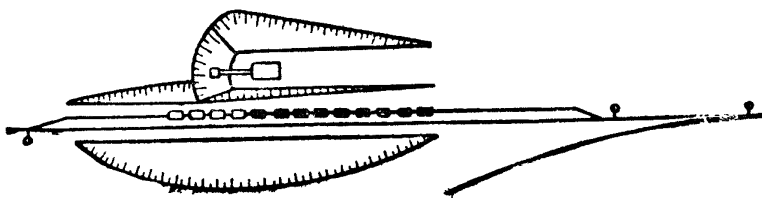
Фиг. 86. Расположение погрузочных путей в „рыбку“
