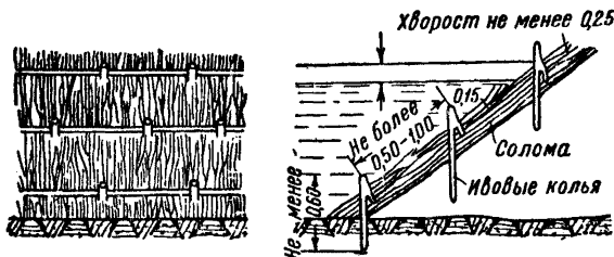
Фиг. 133. Хвостяная выстилка
