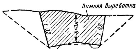
Фиг. 150. Схема разработки выемок глубиной до 3 м в устойчивых грунтах в зимнее время
