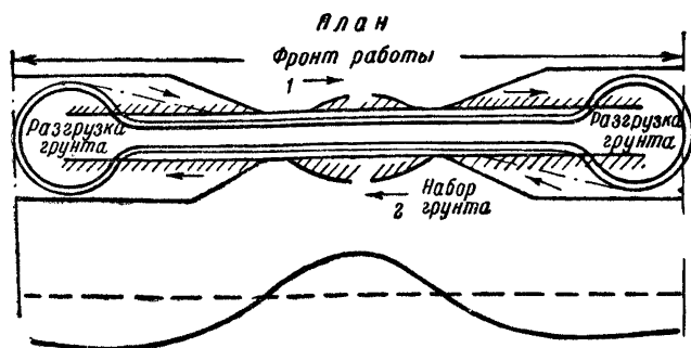
Фиг. 97. Схема движения скреперных поездов по прямой с разворотами 1—начало первого рейса поезда и конец второго рейса; 2—конец первого рейса поезда и начало второго рейса
