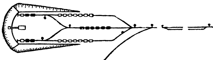
Фиг. 89. Схема расположения погрузочных путей при лобовой разработке выемки
