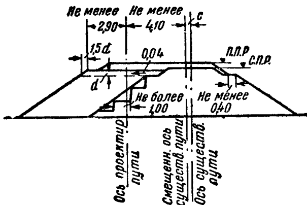
Фиг. 52. Поперечный профиль насыпи второго пути с незначительной разностью уровней первого и второго путей Примечание. d — высота дренирующего слоя; c — расстояние между осью существующего и смещённого первого пути
