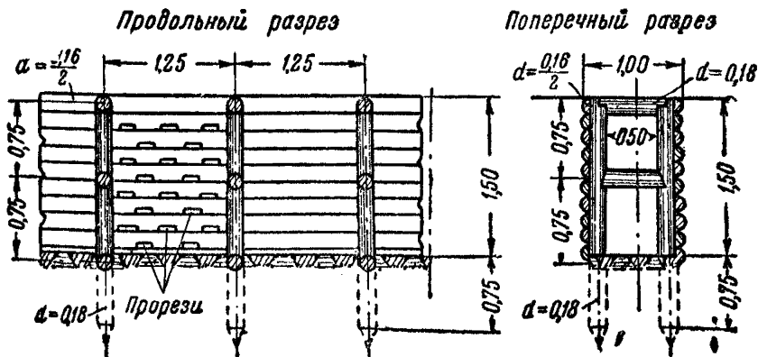
Фиг. 20. Деревянный лоток свайной конструкции глубиной 1,50 м
