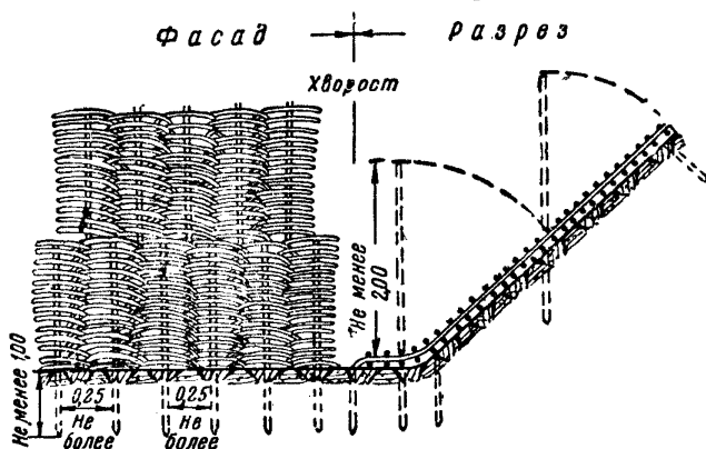
Фиг. 134. Плетнёвое покрытие
