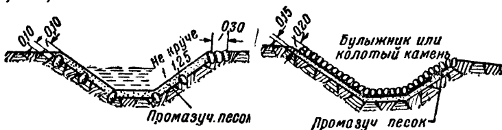
Фиг. 147. Укрепление канав от инфильтрации воды
