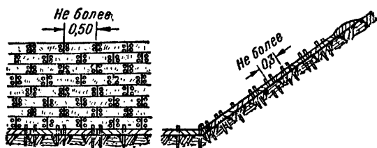
Фиг. 124. Сплошная дерновка плашмя
