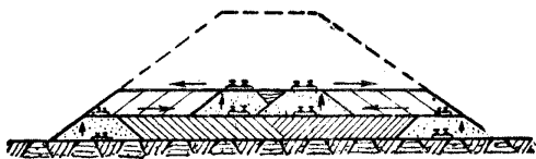
Фиг. 42. Схема возведения насыпи с двух передвигаемых рельсовых путей
