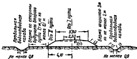
Фиг. 1. Насыпи без резервов высотой 1 м.
