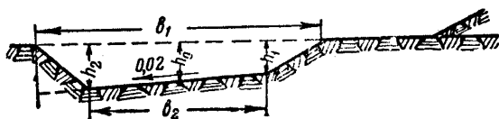
Фиг. 151. Поперечное сечение одностороннего резерва
