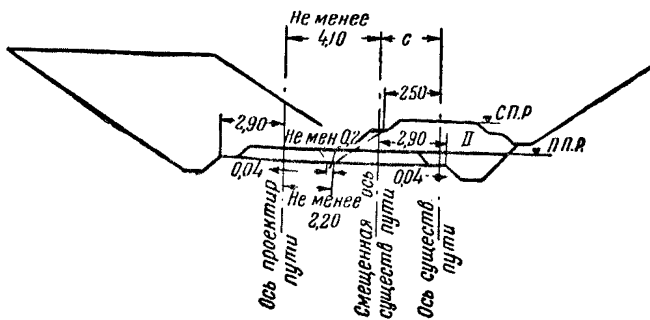
Фиг. 55. Схема разработки выемки второго пути со смещением оси существующего пути
