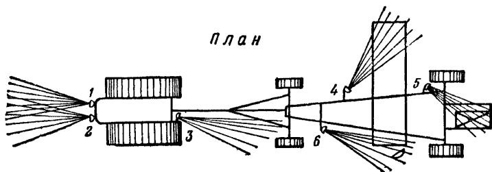
Фиг. 99. Размещение осветительных точек на тракторе и грейдер-элеваторе
