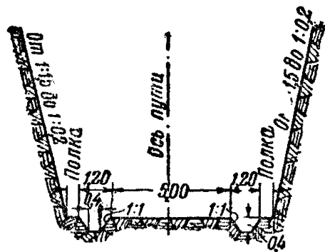
Фиг. 12. Выемка в легковыветривающейся скале
