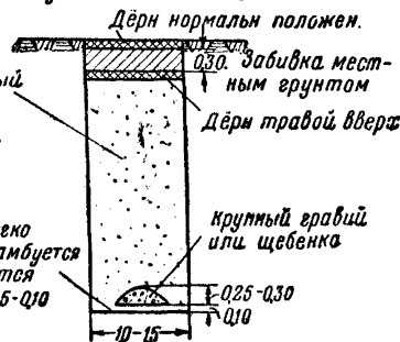
Фиг. 30. Типы заполнений дренажных прорезей
