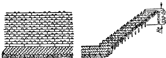
Фиг. 125. Дерновка в стенку
