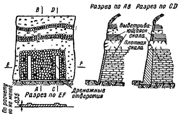
Фиг. 144. Одевающие стенки
