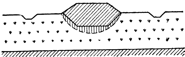
Фиг 61. Схема возведения насыпи высотой менее 3 м на болотах первого типа
