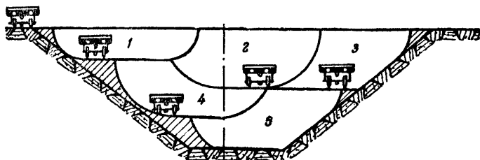
Фиг. 78. Схема разработки выемки с применением пионерной траншеи
