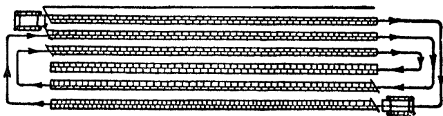
Фиг. 100. Схема проходов бульдозёра при разравнивании грунта, выгруженного из транспортных средств, а также из тракторных скреперов с поперечным перемещением грунта
