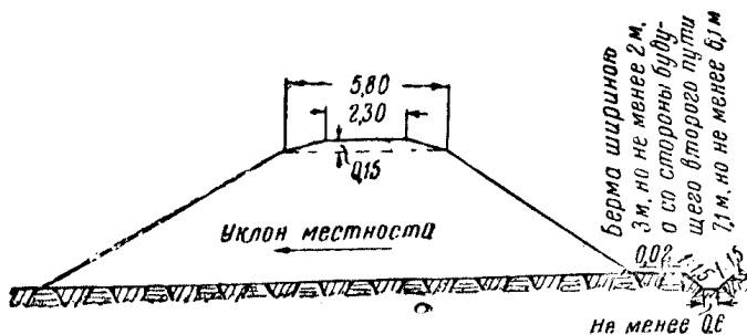
Фиг. 5. Насыпи на пологом косогоре
