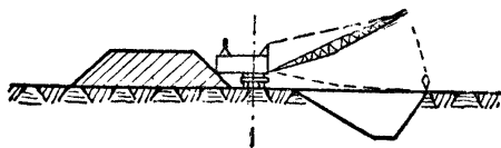
Фиг. 82. Разработка выемки драглайном при одностороннем отвале грунта
