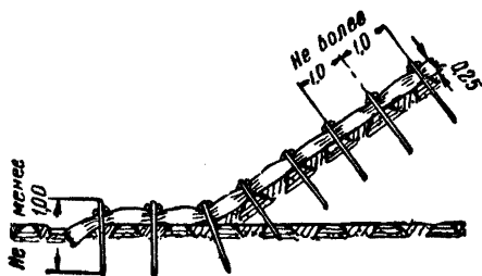
Фиг. 137. Укладка фашин плашмя
