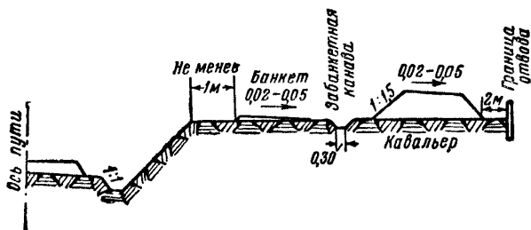
Фиг. 16. Забанкетная канава
