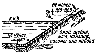
Фиг. 126. Одиночное мощение
