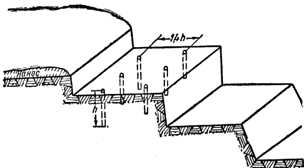
Фиг. 105. Расположение вертикальных шпуров
