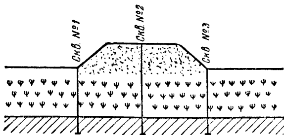
Фиг. 74. Расположение скважин для насыпи новой железнодорожной линии
