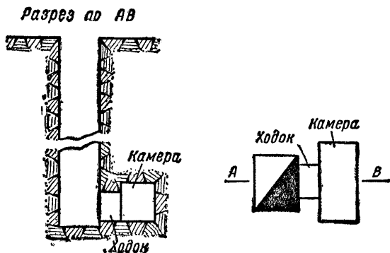
Фиг. 111. Разрез минного колодца с ходком
