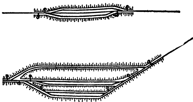
Фиг. 93. Разъездная схема отвальных путей
