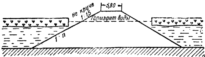
Фиг. 67. Схема возведения насыпи на болотах третьего типа с удалением торфяной корки
