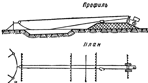
Фиг. 104. Схема возведения насыпи из резерва при помощи передвижной канатно-скреперной установки
