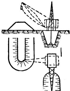
Фиг. 83. Разработка выемки драглайном при отвале грунта в обе стороны
