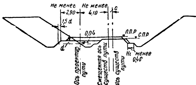
Фиг. 53. Поперечный профиль выемки второго пути с незначительной разностью уровней первого и второго путей
