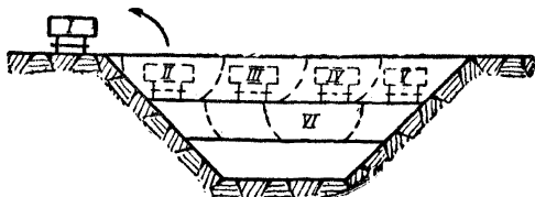
Фиг. 47. Схемы разработки выемки по ширине её
