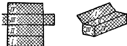
Фиг. 141. Установка габионов
