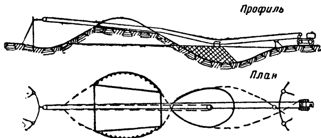
Фиг. 103. Схема разработки выемки канатно-скреперной установкой
