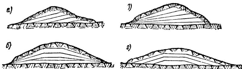
Фиг. 77. Схематические профили расположения забоев в продольном направлении:
