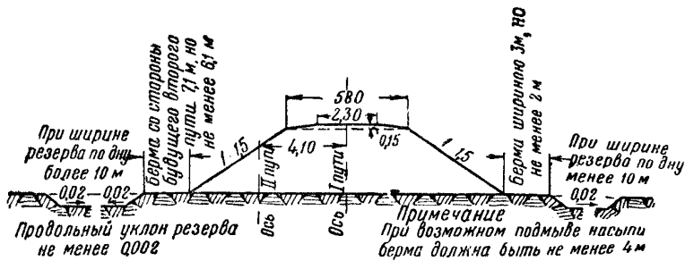
Фиг. 2. Насыпи с резервами при высоте и грунтах, допускающих полуторные откосы
