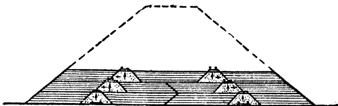
Фиг. 44. Схема отсыпки насыпи с двух путей без передвижки
