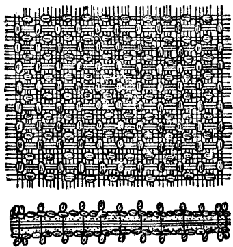
Фиг. 139. Фашинный тюфяк по углам сетки запускают плетни.
