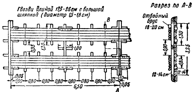
Фиг. 36. Конструкция автолежневой дороги
