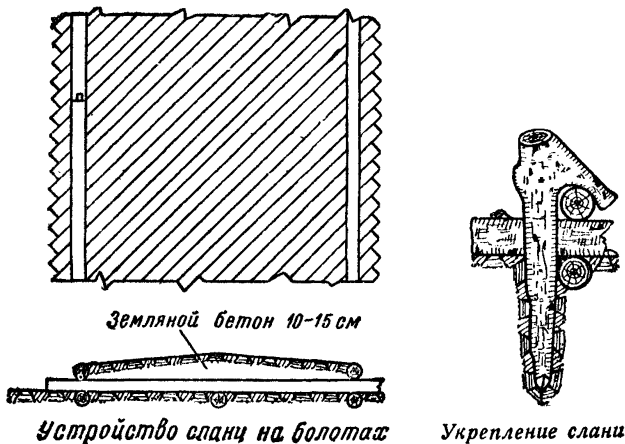
Фиг. 34. Устройство временки на сланях
