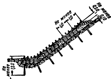
Фиг. 131. Укрепление плетнёвыми клетками
