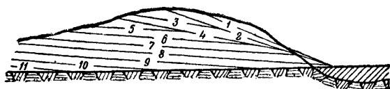
Фиг. 46. Схема разработки выемки последовательными (по высоте) слоями
