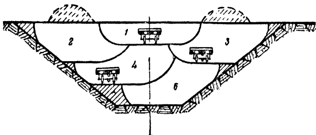
Фиг. 79. Схема разработки пионерной траншеи с отвалом грунта на верх последующих проходок.
