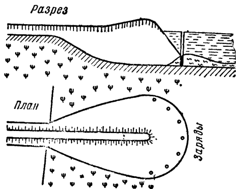
Фиг. 69. Схема расположения зарядов для удаления болотных образований взрывным способом
