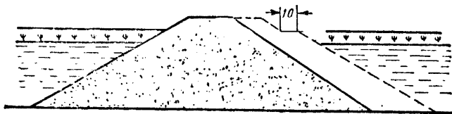
Фиг. 73. Схематический профиль присыпки второго пути на болотах третьего типа
