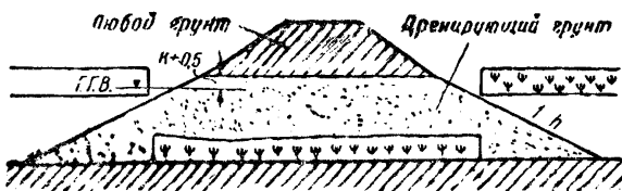
Фиг. 70. Схема отсыпки насыпи на болотах с погружением торфяной корки
