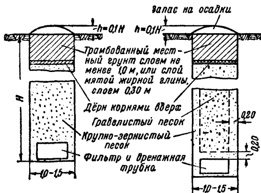
Фиг. 31. Заполнение дренажной прорези при понижении уровня грунтовых вод
