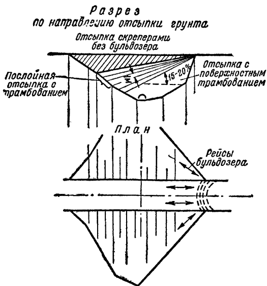
Фиг. 101. Схема работы бульдозёра по засыпке глубоких оврагов.
