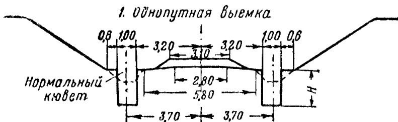
Фиг. 18. Расположение продольных лотков в выемках—однопутная выемка
