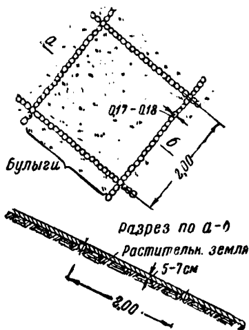
Фиг. 122. Ленты из камня
