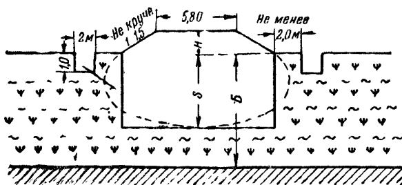
Фиг. 66. Схема возведения насыпи на болотах второго типа глубиной более 3 м
