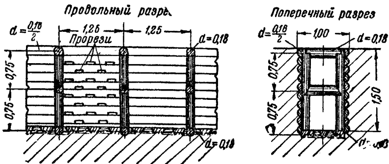
Фиг. 23. Деревянный лоток рамной конструкции глубиной 1,50 м
