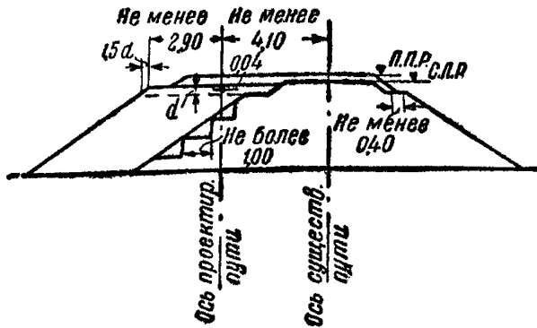
Фиг. 50. Поперечный профиль присыпки второго пути без смещения оси пути Примечание. d — высота дренирующего слоя.
