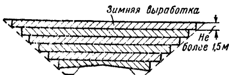
Фиг. 149. Схема разработки выемки глубиной более 3 м в зимнее время
