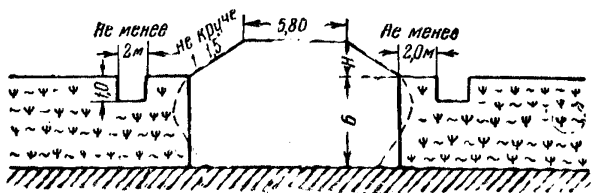
Фиг. 65. Схема возведения насыпи на болотах второго типа глубиной менее 3 м
