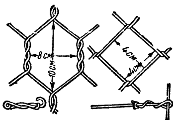
Фиг. 140. Габионная сетка
