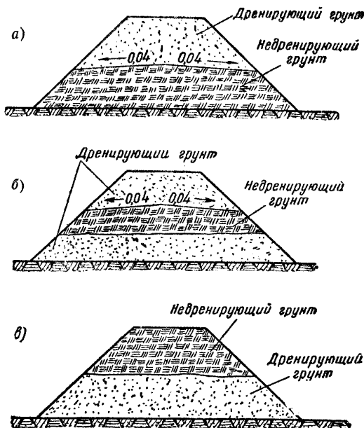
Фиг. 37. Схема допустимого расположения грунтов в теле насыпи
