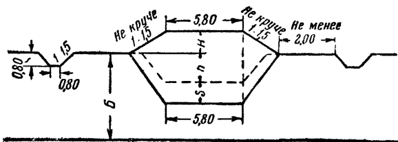
Фиг. 62. Схематический профиль насыпи высотой менее 3 м на болотах первого типа для подсчёта объёмов земляных работ и выторфовывания
