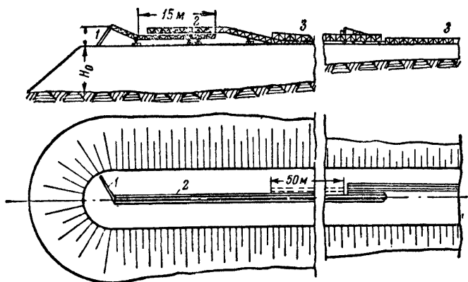
Фиг. 91. Расположение телескопического транспортёра рядом с основным транспортёром 1, 2, 3—номера транспортёров
