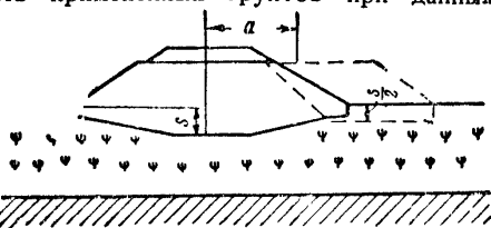
Фиг. 72. Схематический профиль присыпки второго пути на болотах второго типа
