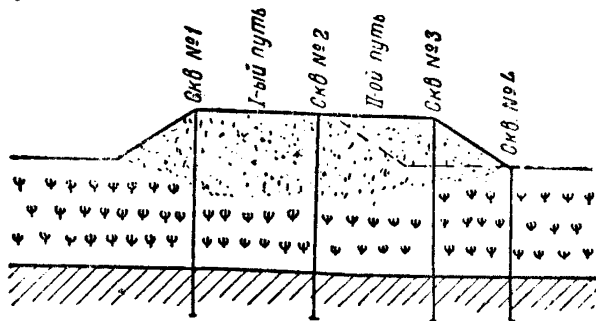
Фиг. 75. Расположение скважин при присыпке второго пути
