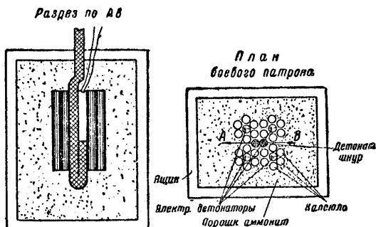
Фиг. 114. Схема боевика
