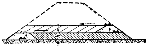
Фиг. 41. Схема возведения насыпи с одного передвигаемого рельсового пути
