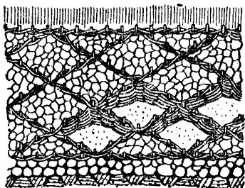
Фиг. 130. Укрепление плетнёвыми клетками
