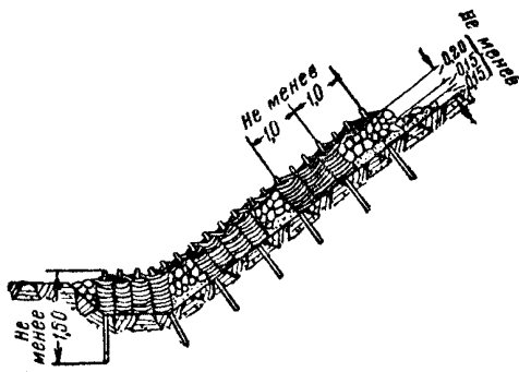
Фиг. 132. Укрепление плетёвыми клетками
