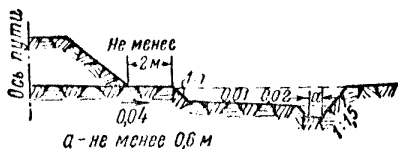
Фиг. 14. Водоотводная канава в резерве
