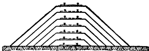
Фиг. 40. Запрещённый способ отсыпки насыпи
