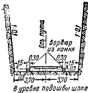
Фиг. 11. Выемка в слабовыветривающейся скале
