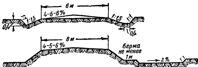
Фиг. 32. Поперечный профиль полотна времянки
