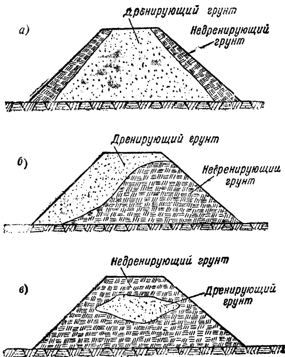
Фиг. 38. Схема недопустимого расположения грунтов в теле насыпи
