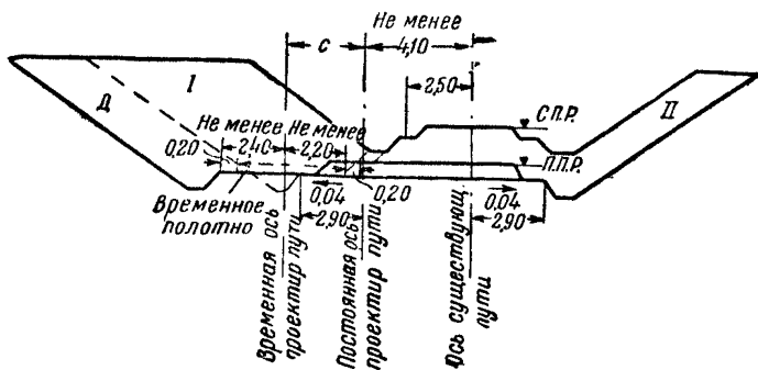
Фиг. 54. Схема разработки выемки второго пути без смещения оси существующего пути
