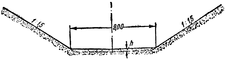
Фиг. 10. Выемка в песчаных грунтах в районах с сухим климатом, обеспеченная полным впитыванием во всякое время года
