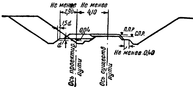
Фиг. 51. Поперечный профиль разработки выемки для второго пути без смещения оси пути
