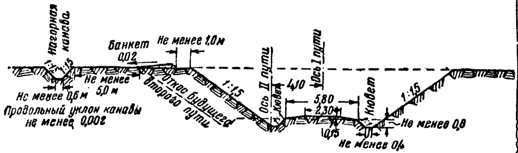
Фиг. 8. Выемка без кавальеров глубиной более 2 м
