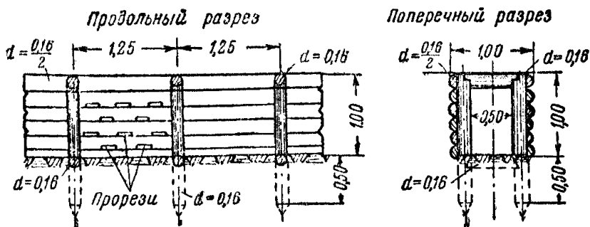
Фиг. 19. Деревянный лоток свайной конструкции глубиной 1,00 м
