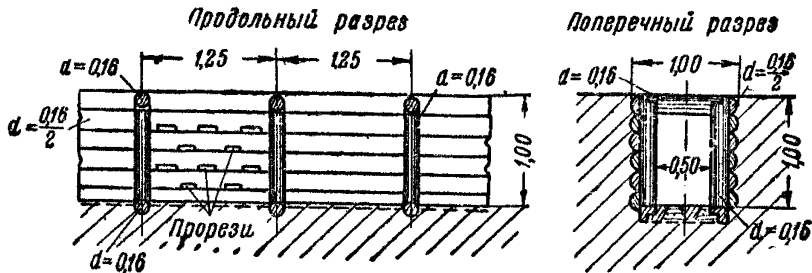
Фиг. 22. Деревянный лоток рамной конструкции глубиной 1,00 м
