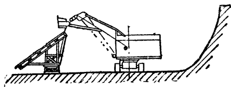
Фиг. 81. Схема разгрузки экскаватора через подвижную наклонную плоскость
