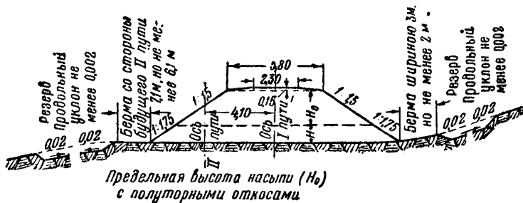
Фиг. 3. Высокие насыпи (до 12 м)
