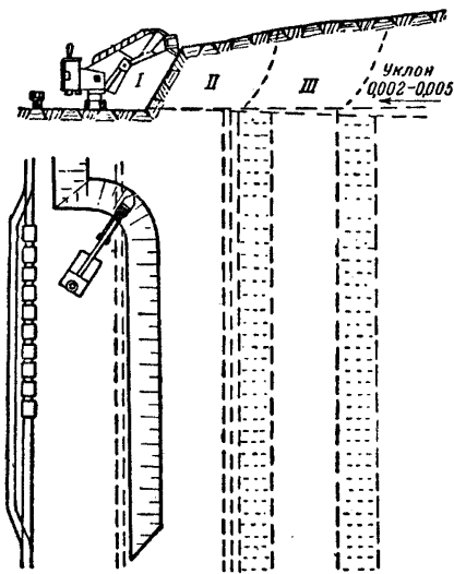
Фиг. 76. Схема продольной разработки открытого массива
