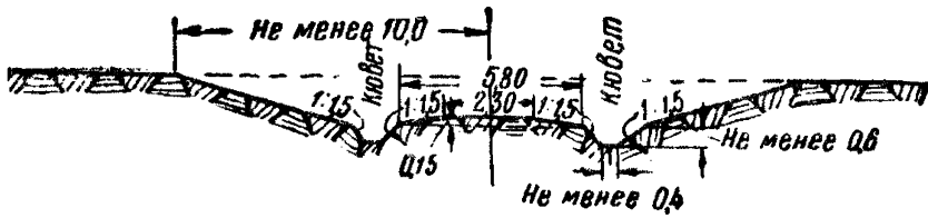
Фиг. 7. Раскрытая выемка без кавальеров глубиной до 2 м.
