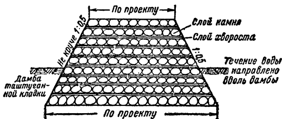
Фиг. 142. Схема таштуганной кладки
