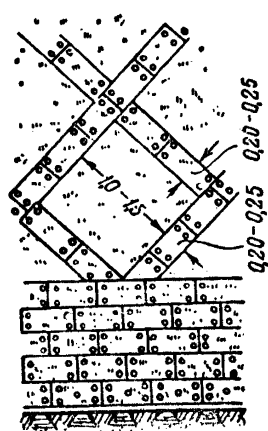
Фиг. 121. Дерновка в клетку
