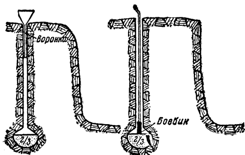
Фиг. 106. Заряжание котловых шпуров
