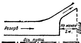
Фиг. 15. Выпуск воды из резерва
