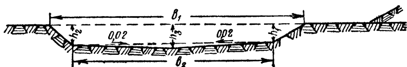
Фиг. 152. Поперечное сечение двустороннего резерва
