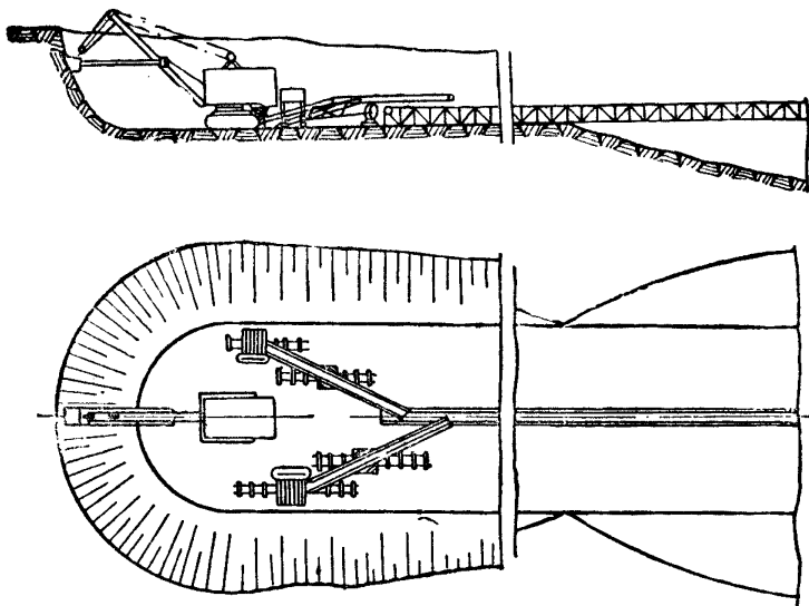
Фиг. 90. Схема разработки выемки прямой лопатой с погрузкой грунта через подвижные лёгкие транспортёры 15 м длиной на магистральный ленточный транспортёр
