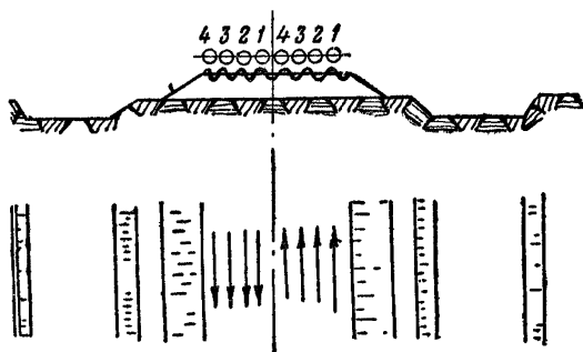
Фиг. 102. Схема работы бульдозёра при разравнивании грунта, отсыпаемого грейдер-элеватором (поперечный разрез и план)
