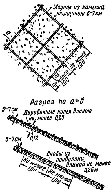
Фиг. 123. Ленты из камышёвых жгутов
