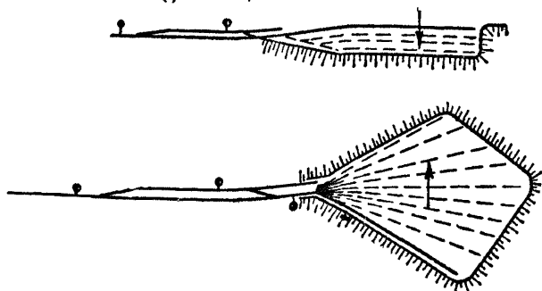
Фиг. 92. Схема расположения тупиковых отвальных путей
