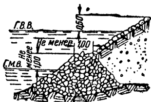
Фиг. 128. Каменная наброска — контрбанкет
