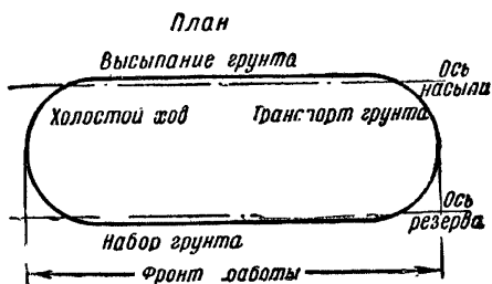
Фиг. 95. Схема движения скреперных поездов по эллипсу
