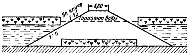
Фиг. 68. Схема возведения насыпи на болотах третьего типа без удаления торфяной корки
