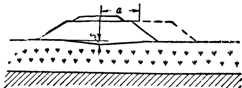
Фиг. 71. Схематический профиль присыпки второго пути на болотах первого типа
