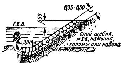
Фиг. 127. Двойное мощение
