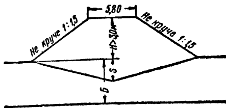
Фиг. 60. Схематический профиль насыпи высотой 3 м и более на болотах первого типа для подсчёта объёмов земляных работ
