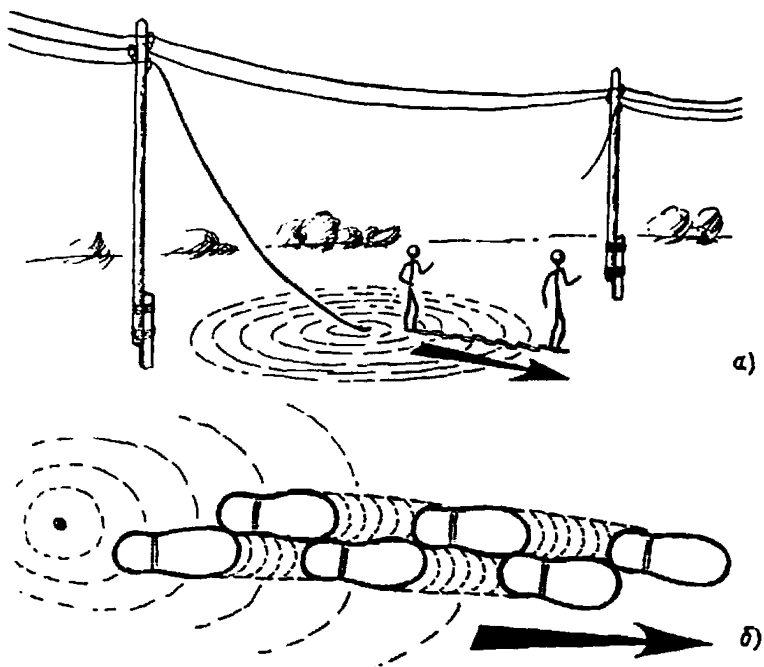
Рис. 7. Правильное перемещение в зоне растекания тока замыкания на землю: а — удаление от точки замыкания на землю токоведущей части; б — следы с обуви
