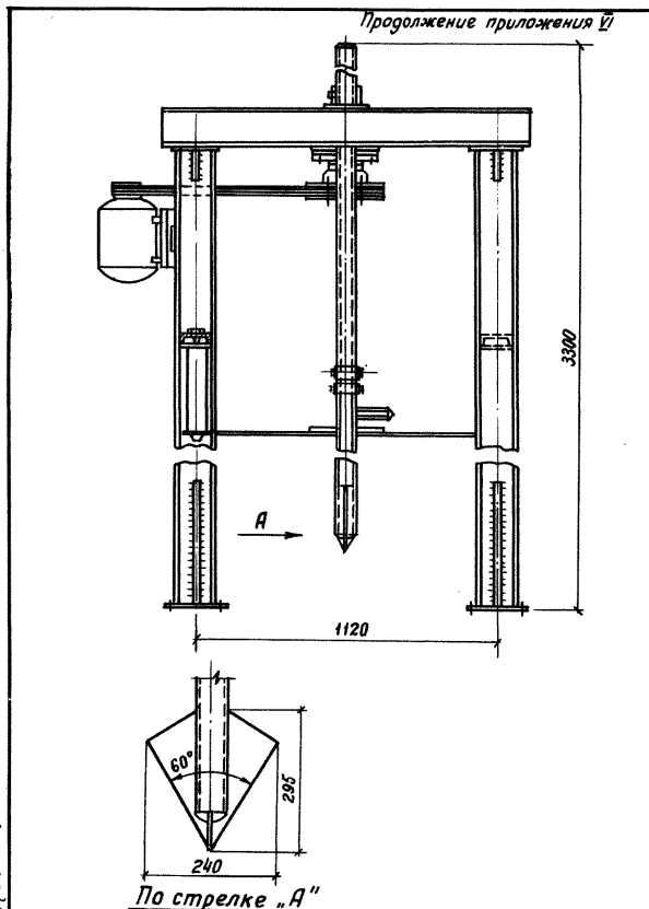
Рис. 25. Устройство по механизированной разгрузке твердых реагентов в расходные чаны (по материалам березовской обогащательной фабрики)
