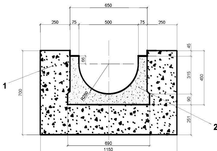
1 – закрытый лоток; 2 – обойма омоноличивания лотка
