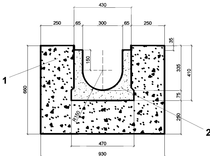
Рисунок В.1 - Поперечное сечение обоймы омоноличивания лотка шириной 300 мм
