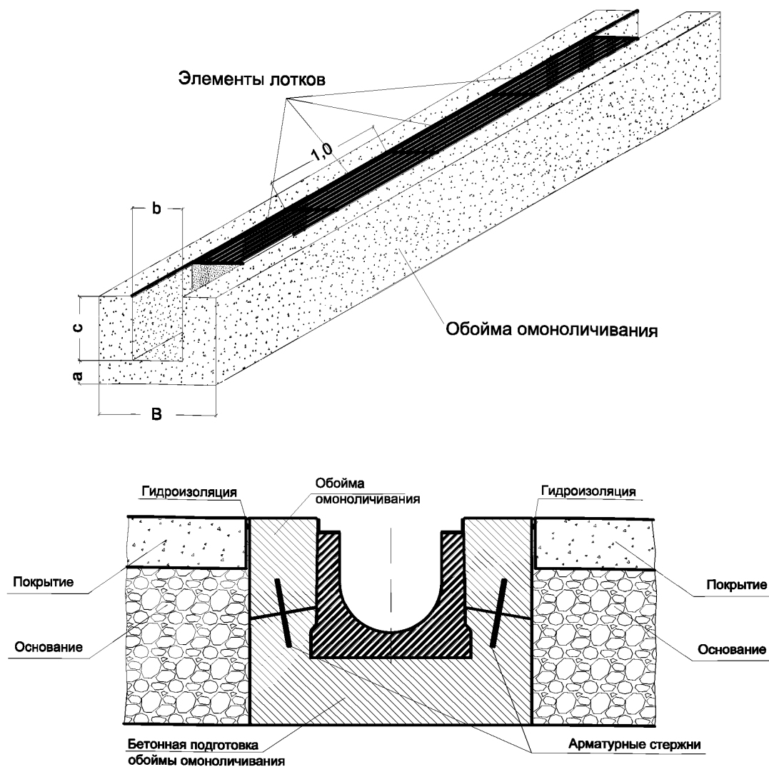
Рисунок 2 - Конструкция монтажа лотка закрытого типа в обойму омоноличивания
