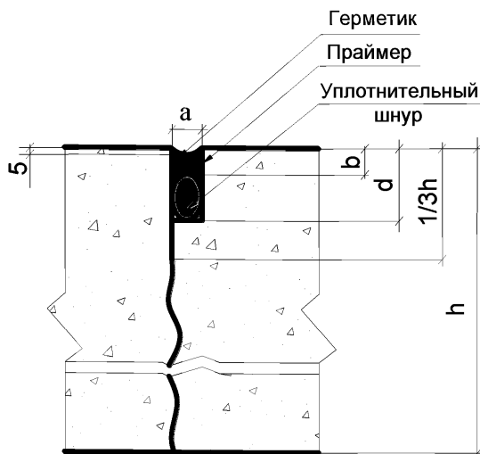
Рисунок 4 - Деформационный шов сжатия
