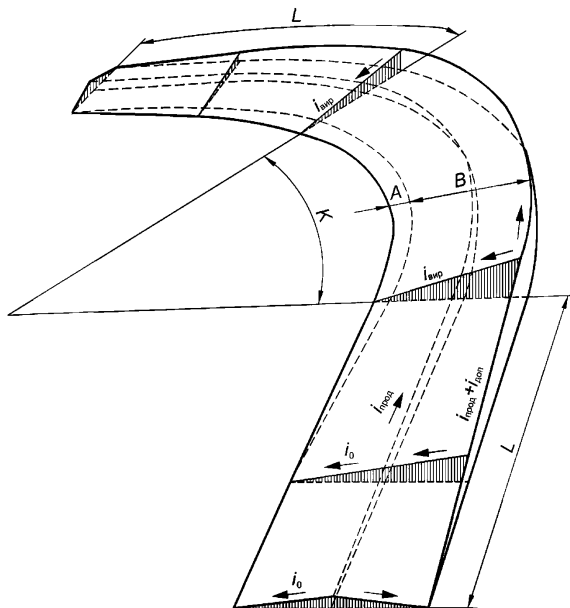
Рисунок 27 – Схема виража на дороге с двухскатной проезжей частью
