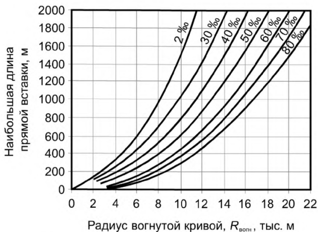
Рисунок 41 – Наибольшая длина прямой вставки между двумя вертикальными кривыми на дорогах I технической категории. Цифры на кривых (20-80 ‰) – алгебраическая разность уклона прямой вставки и точки стояния
