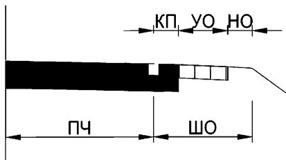
Рисунок 8 – основные элементы обочины: КП – краевая полоса; УО – укрепленная часть обочины; НО – неукрепленная часть обочины; ШО – общая ширина обочины; ПЧ – проезжая часть.
