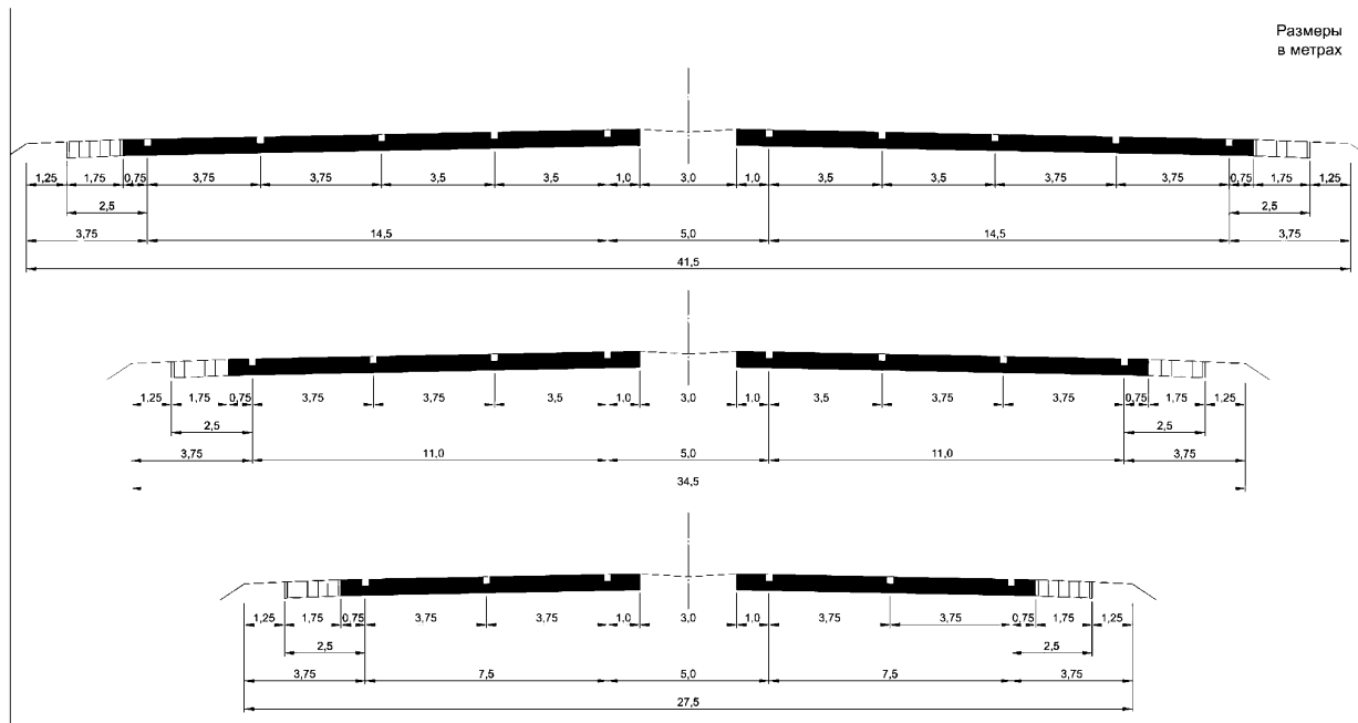
Рисунок 11 – Типовые поперечные профили дорог категории IА для расчетной скорости – 60-120 км/ч с ограждением (конструкция ограждения показана условно)
