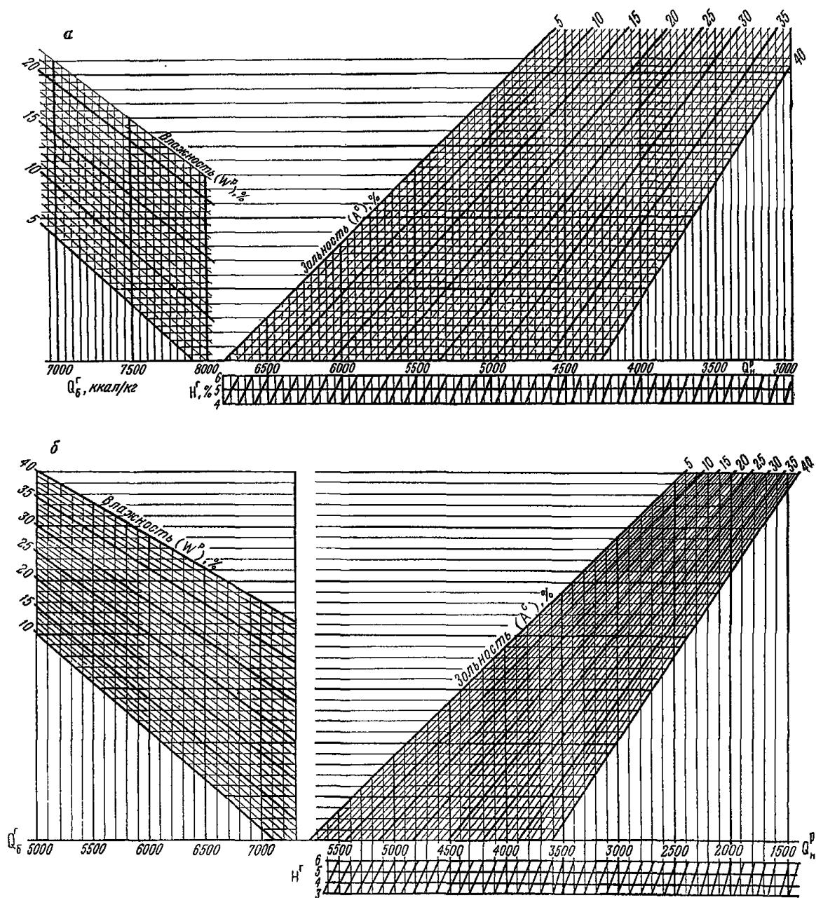
Рис. 10. Номограмма для расчета низшей теплоты сгорания рабочего топлива (по Э. М. Паху) а — для Q_g^0 = 7000 ккал/кг; W_p = 5-20\% ; б — для Q_g^0 = 5000-7000 ккал/кг; W_p = 10-40\%
