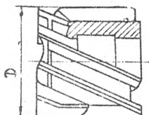
Рис. 29-фреза цилин- дрическая со встав- ными ножами
