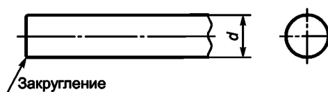
Рисунок 3 — Форма А (конец круглого сечения)
