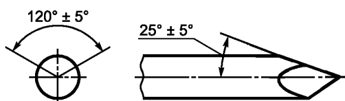
Рисунок 2 — Рекомендуемое острие скелетного штифта Стейнманна
