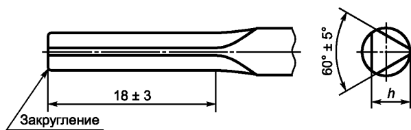
Рисунок 5 — Форма С (конец треугольного сечения)
