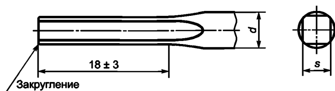
Рисунок 4 — Форма В (конец квадратного сечения)
