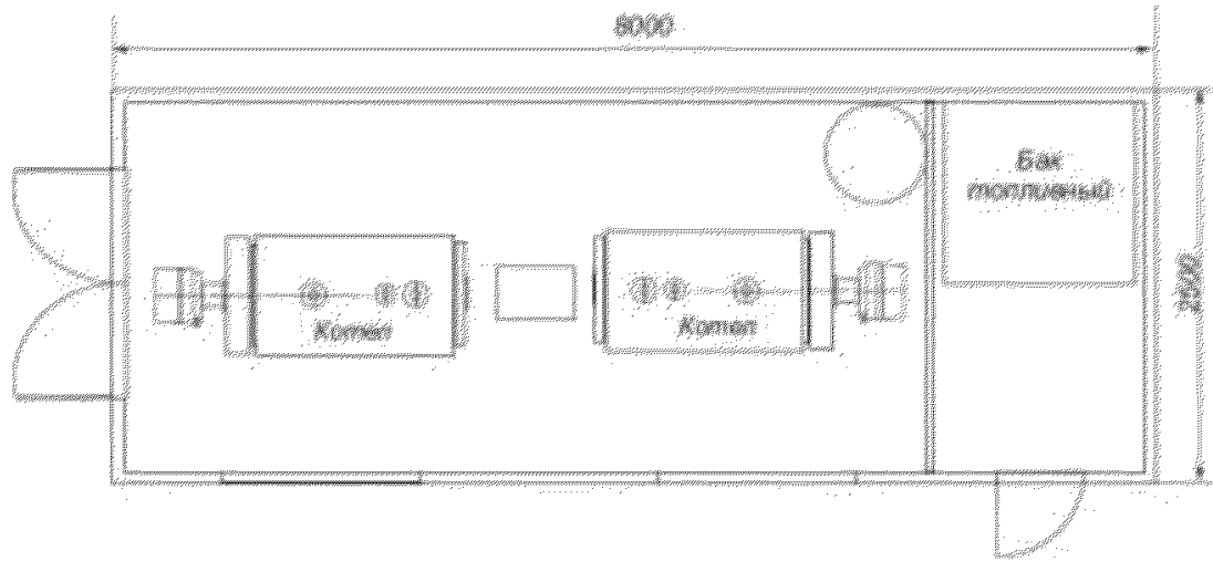
Рисунок 5.2 – Котельная
