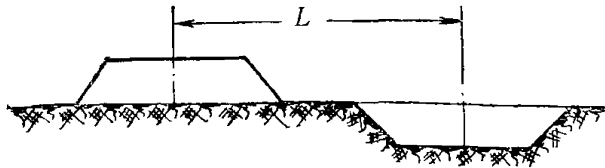
Рис. 2. Расстояние перемещения грунта бульдозером, грейдером и грейдер-элеватором ( L ) равно среднему расстоянию между серединами разрабатываемого и отсыпаемого объемов грунта за учитываемый период.
