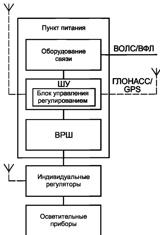
б — схема с блоком управления регулированием
