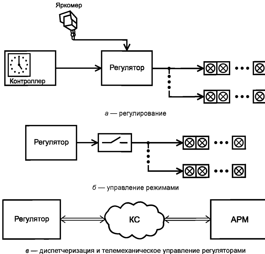
Рисунок 5 — Цепочные структуры телемеханических сетей управления
