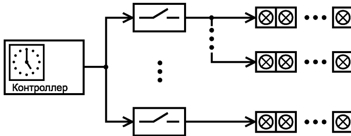
Рисунок 1 — Автоматический режим переключения с учетом времени суток
