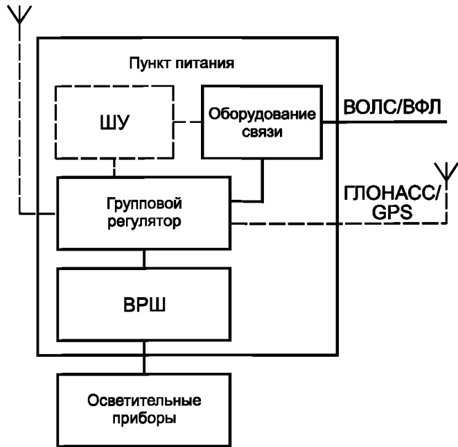
Рисунок 11 — Общая схема подуровня 1Б для группового регулирования
