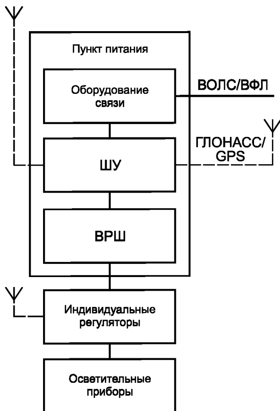
а — схема без блока управления регулированием
