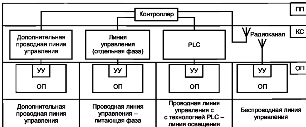
Рисунок 8 — Схема комбинированных каналов связи
