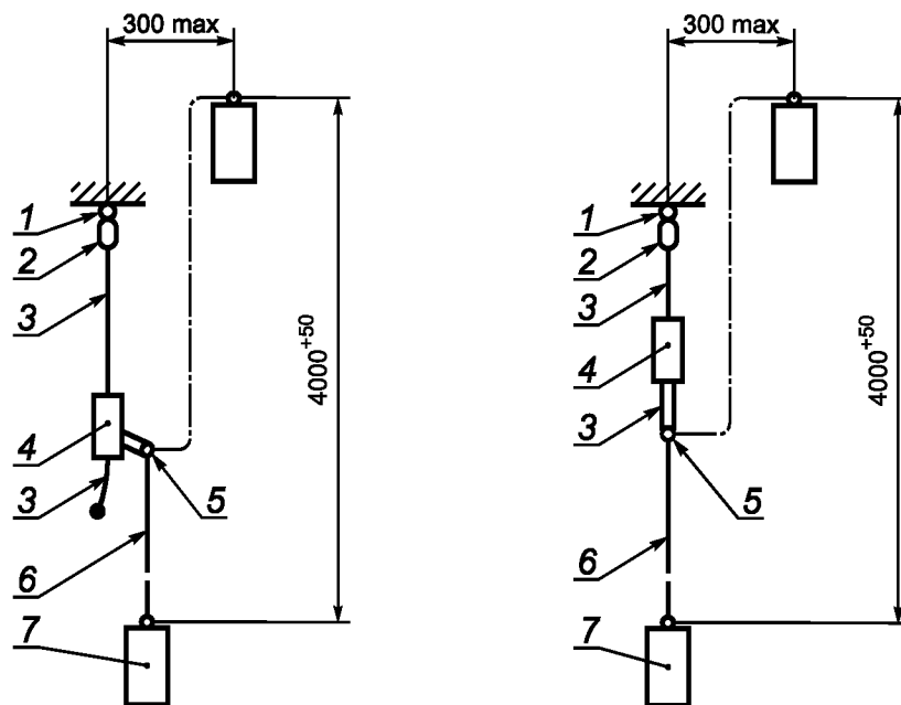
а) Точка соединения находится на устройстве регулирования длины
