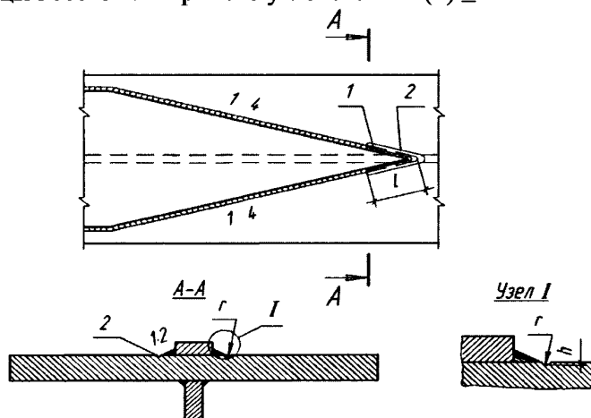
Рисунок 42 – Схема обработки косых угловых швов на конце обрываемого в пролёте поясного листа главной балки с многослойным поясом, а также прямых угловых швов
