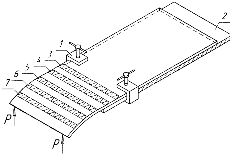
1 – струбины; 2 – стол (стенд); 3 — 7 – полосы нагрева металла; P – нагрузки (усилия домкратов)
