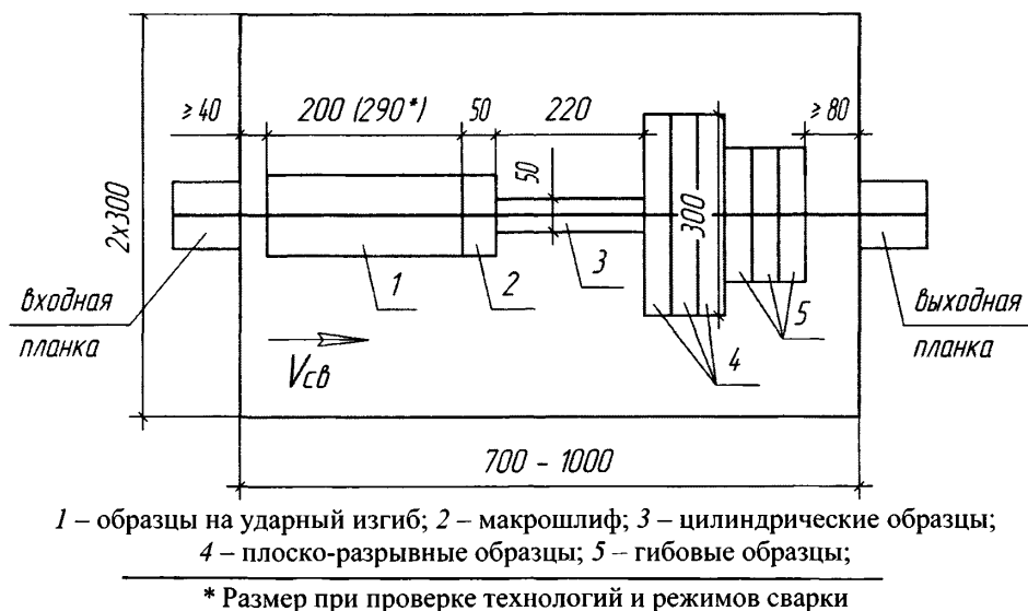
Рисунок Е.6 – Схема вырезки образцов из стыкового соединения
