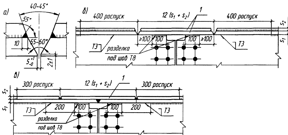
Рисунок 2 – Схемы изменения ширины и толщины элементов балок
