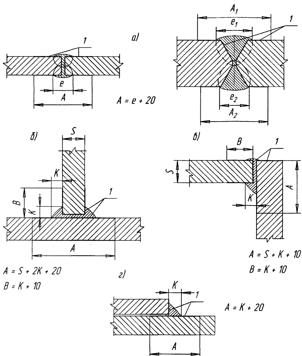
Соединения: а – стыковые; б – тавровые; в – угловые; г – нахлесточные; 1 – зоны зачистки
