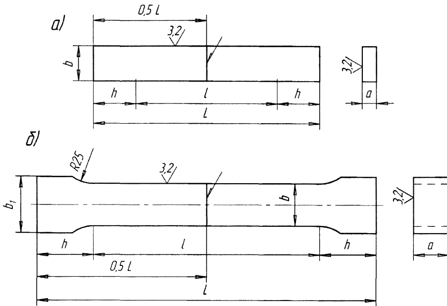
a – образец типа XII; б – образец типа XIII
