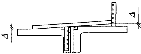
Рисунок 21 – Измерение перекоса двумя угольниками и линейками
