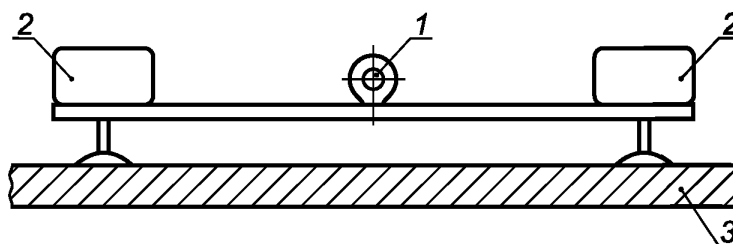
Рисунок 7 — Пример анкерного устройства типа D
