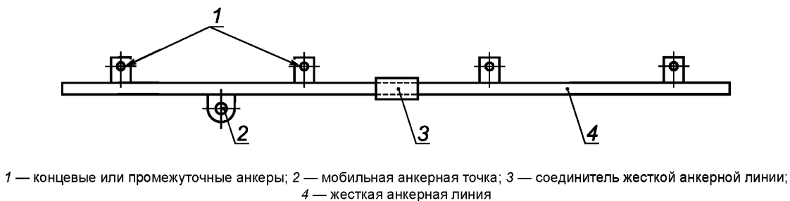
Рисунок 7 — Пример анкерного устройства типа D
