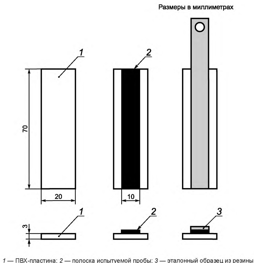
Рисунок С.2 — Подготовка испытуемой пробы
