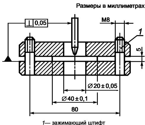
Рисунок 9— Удерживающее устройство
